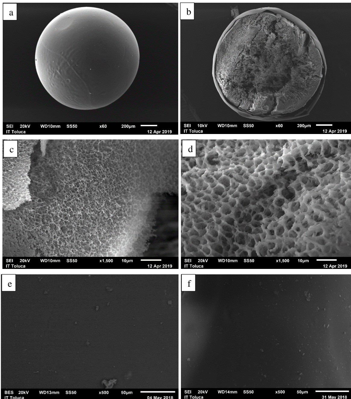
Figura 3.4 Micrografías del hidrogel Q-TPP a) esfera completa S-IRR a 60X b) esfera IRR seccionada a 60X c) acercamiento del interior de la esfera IRR a 1500X d) acercamiento del interior de la esfera S-IRR a 1500X e) superficie de la esfera S-IRR a 500X f) superficie de la esfera IRR a 500X
