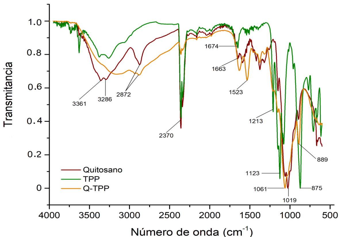
Figura 3.6 Comparación de los espectros del quitosano (Q), tripolifosfato de sodio (TPP) y el hidrogel Q-TPP
