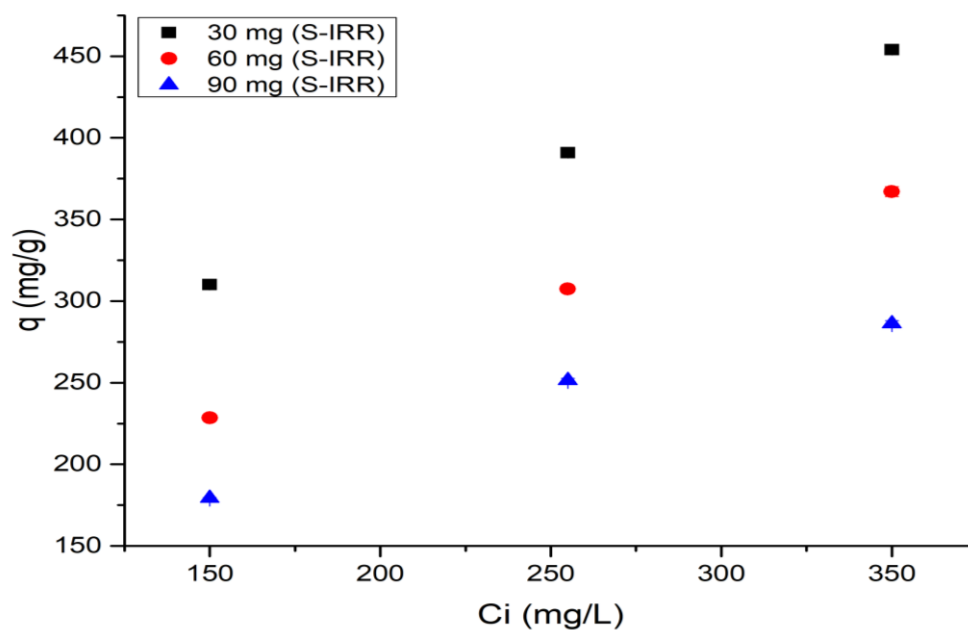
Figura 3.13 Gráfica de la prueba de efecto de la masa del hidrogel S-IRR en la capacidad de adsorción del colorante RJ2.
