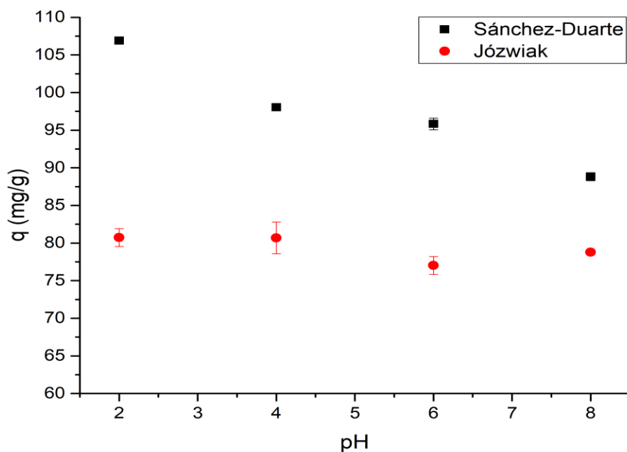
Figura 3.2 Comparación del efecto de pH en las capacidades de adsorción del colorante RJ2 utilizando los hidrogel Q-TPP sintetizados por diferentes metodologías
