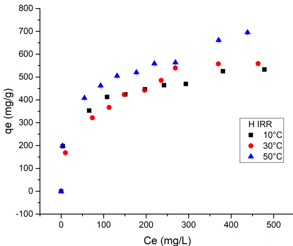
Figura 3.26 Gráfica de la isoterma de adsorción del colorante RJ2 10,30 y 50°C del hidrogel Q-TPP IRR
