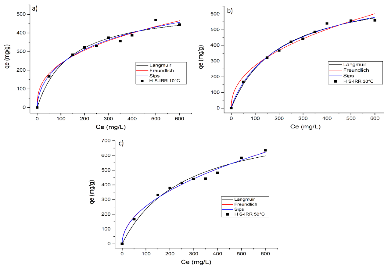
Figura 3.27 Ajuste de los datos experimentales de las isotermas de adsorción de RJ2 con el hidrogel Q-TPP S-IRR a los modelos de Langmuir, Freundlich y Sips a a) 10°C, b) 30°C y c) 50°C
