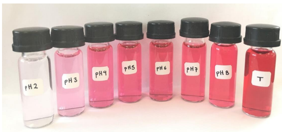
Figura 3.12 Soluciones residuales de la adsorción del colorante respecto al efecto de pH de la solución con el hidrogel Q-TPP S-IRR
