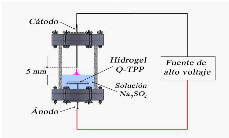
Figura 2.2 Reactor de plasma de descarga luminiscente
