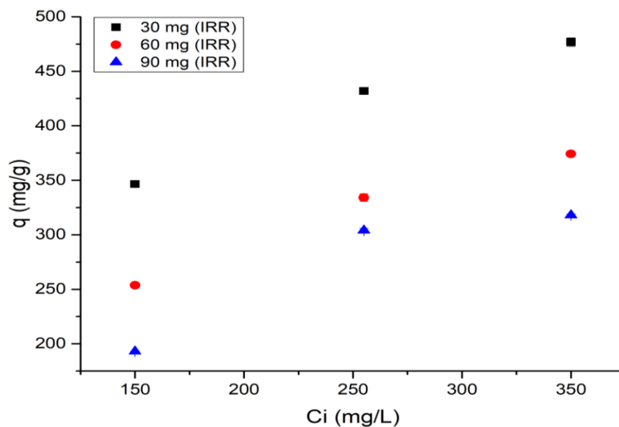
Figura 3.20 Gráfica de la prueba de efecto de la masa del hidrogel IRR en la capacidad de adsorción del colorante RJ2.
