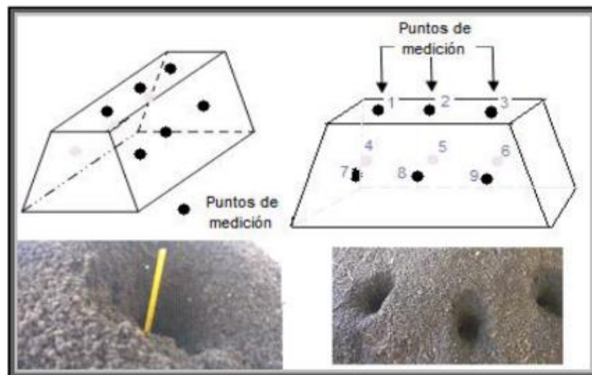
Figura 3.3 Puntos estratégicos de medición de temperatura
