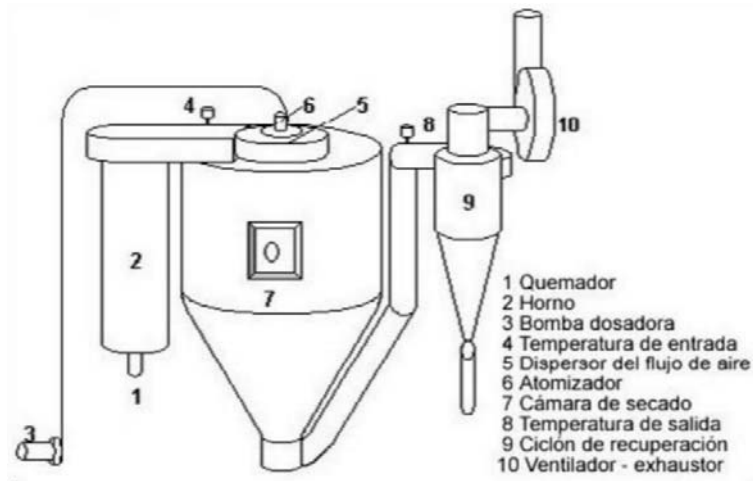
Figura 1.28 Partes de un secador por aspersion (Sprayprocess, 2016)
