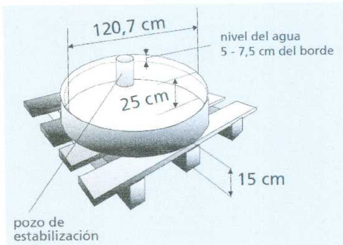
Figura 11. Tanque evaporimetro tipo A
