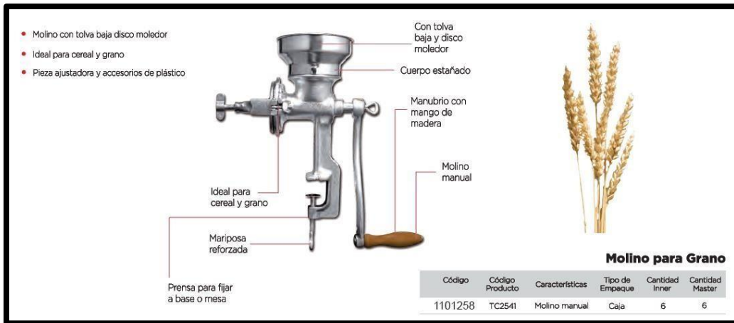
Figura 2.3 Molino para grano, marca TOOLCRAFT.
