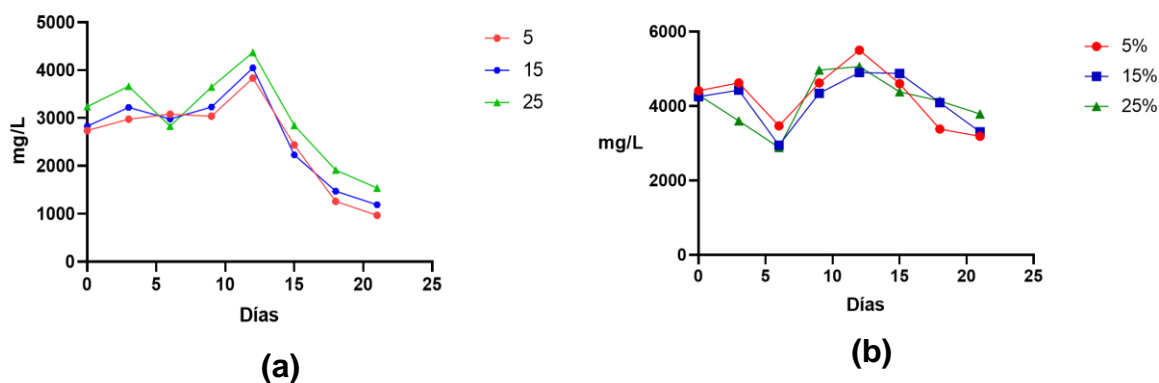
Figura 3.3.5 SST de N. oculata en ARA
