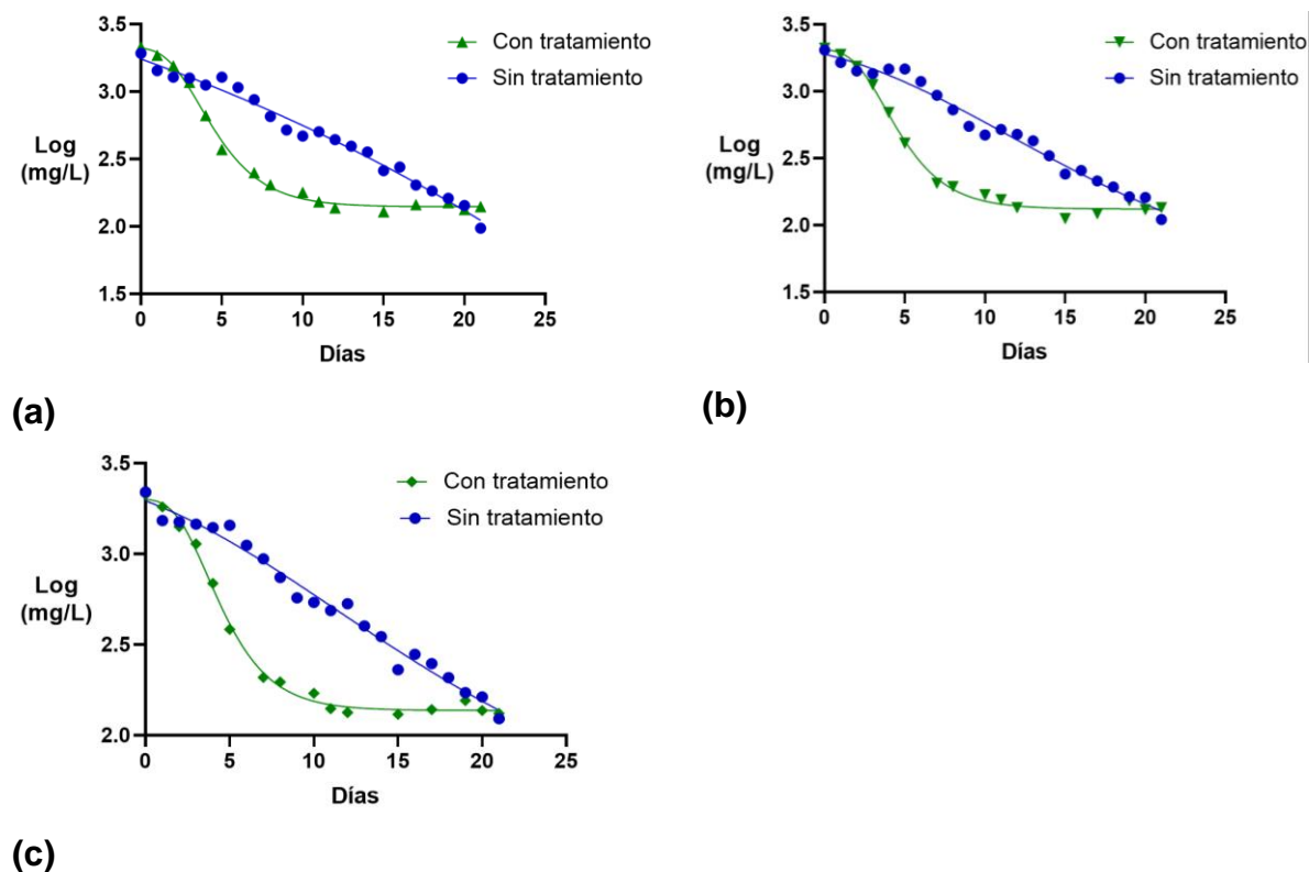
Figura 3.4.2. Remoción de la DQO soluble evaluado en las 3 concentraciones e inóculo: a) 5 % v/v, b) 15 % v/v y c) 25 % v/v.
