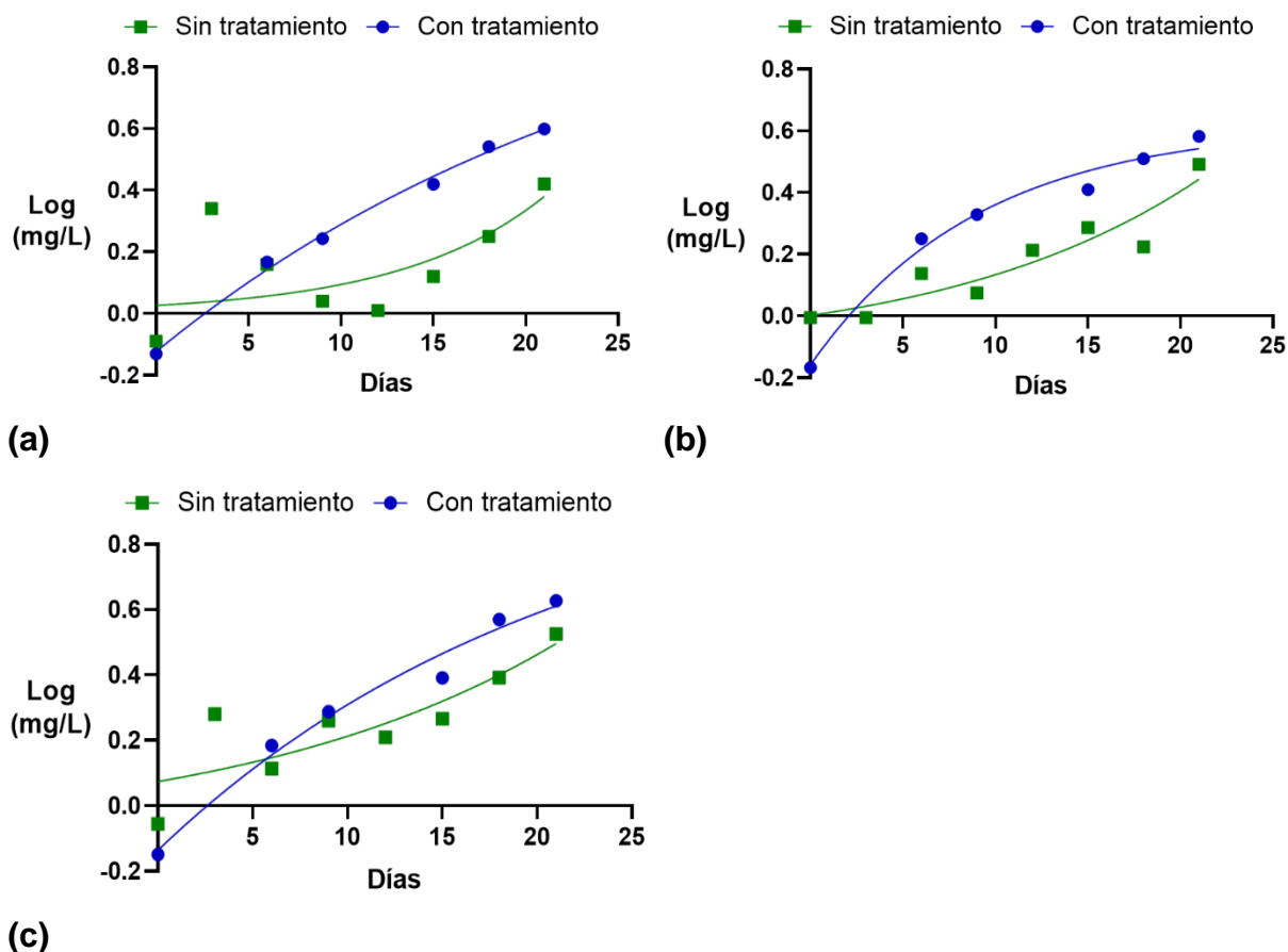
Figura 3.4.5. Generación de biomasa microalgal evaluada en las 3 concentraciones e inóculo: a) 5 % v/v, b) 15 % v/v y c) 25 % v/v.
