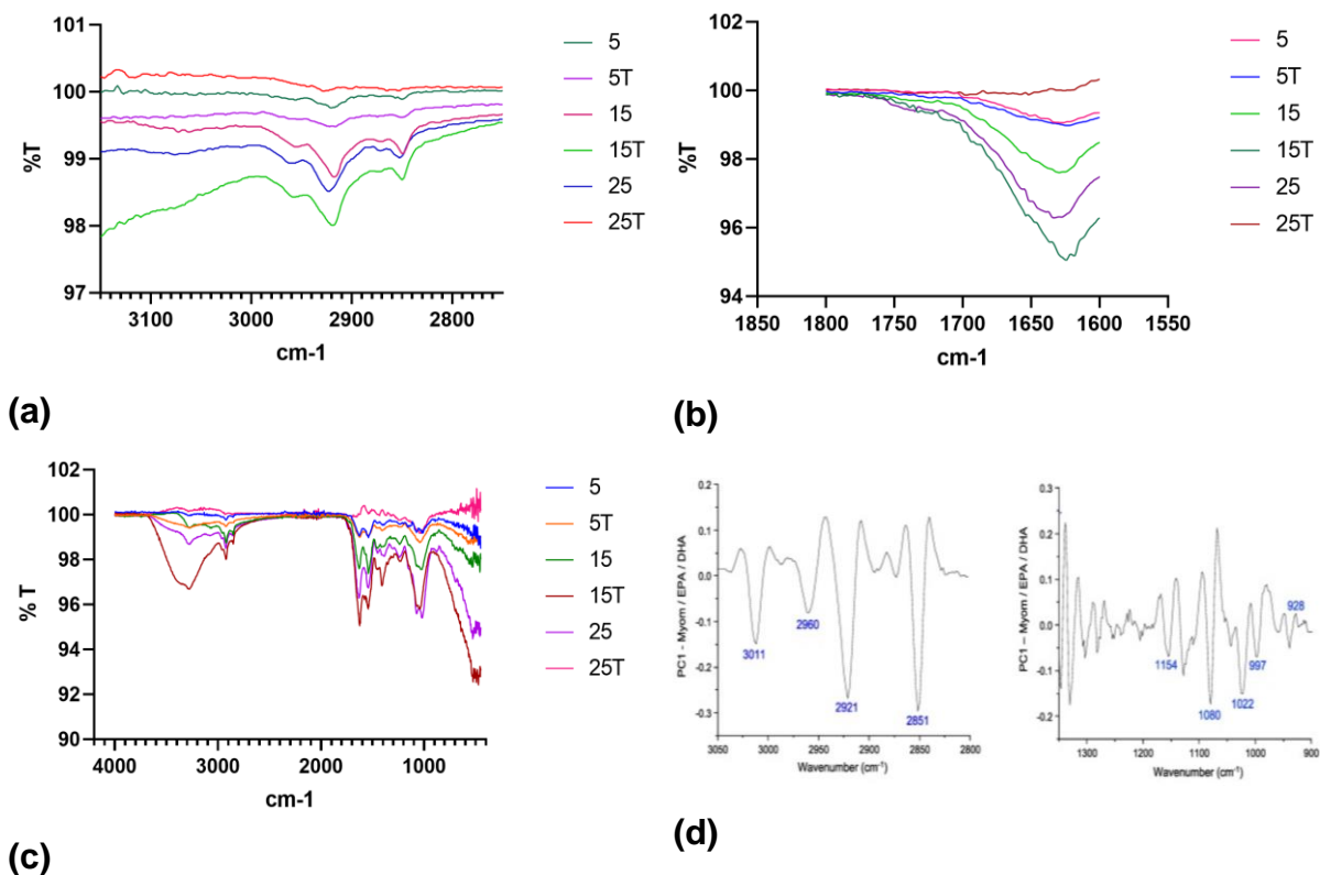
Figura 3.7 Perfil de AGP de la biomasa en FTIR
