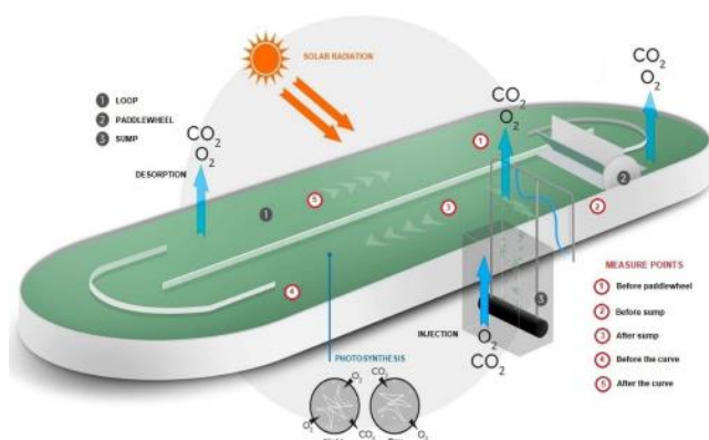
Figura 1.8 Fotobiorreactor abierto tipo raceway
