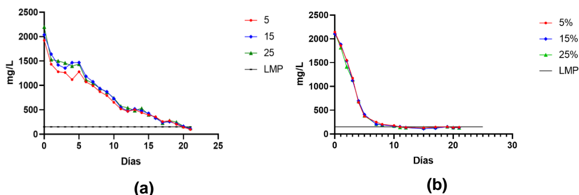
Figura 3.3.8 DQO soluble en ARA
