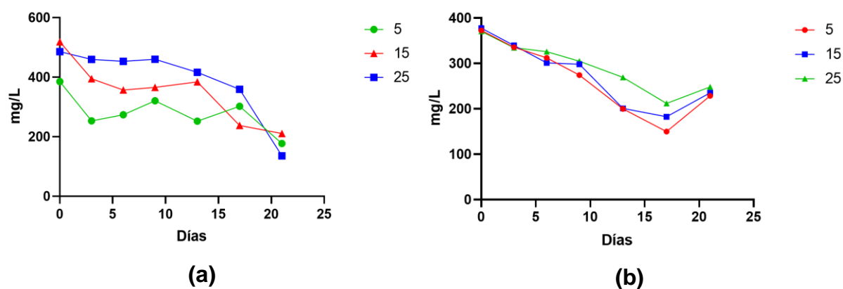
Figura 3.3.10 Remoción de fósforo total en ARA
