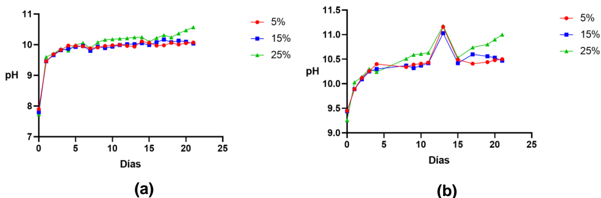
Figura 3.3.2 Comportamiento del pH en ARA
