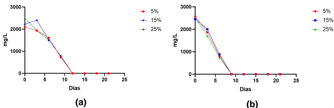
Figura 3.3.9 Remoción del nitrógeno en ARA
