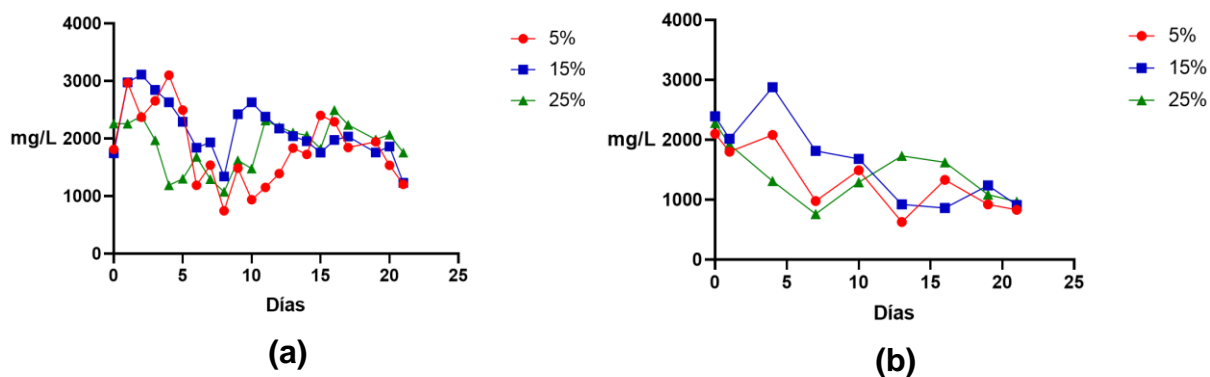
Figura 3.3.4 Comportamiento de los STV en ARA con N. oculata
