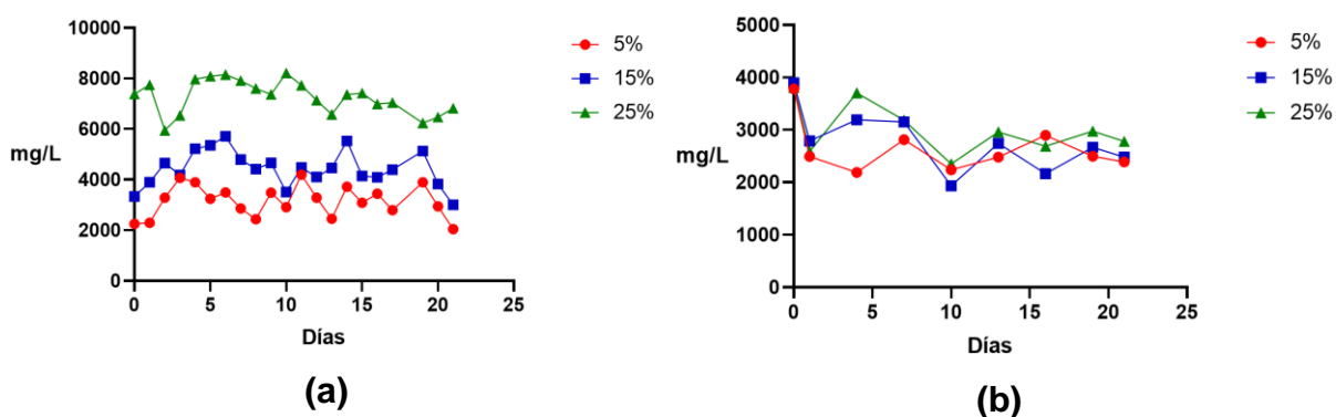
Figura 3.3.3 Comportamiento de los ST en ARA con N. oculata
