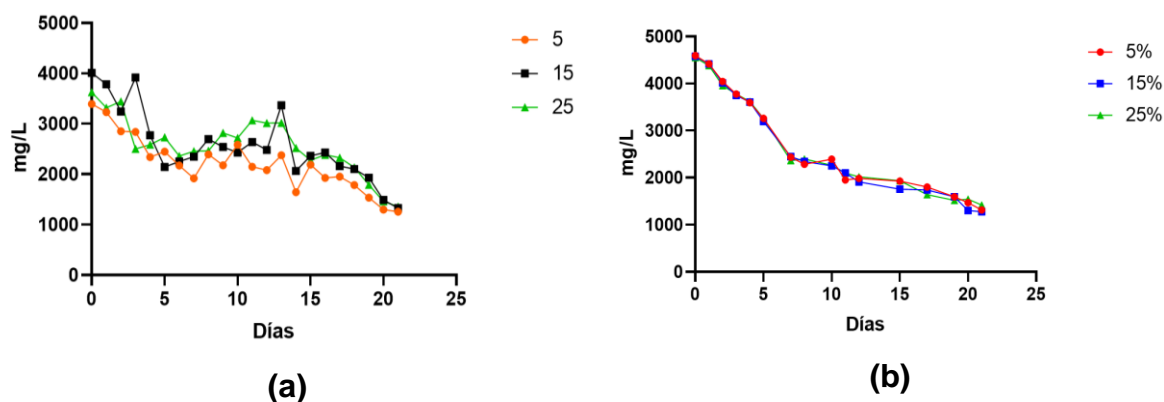
Figura 3.3.6 DQO de N. oculata en ARA
