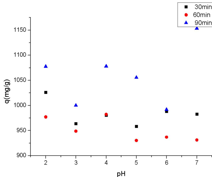
Figura 3.14 Efecto del pH sobre la capacidad de adsorción de la solución con esferas modificadas por plasma a tres diferentes tiempos (esfera de 3.1 mm Ø).
