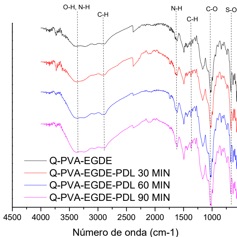
Figura 3.5 Espectro de las esferas de 3.1 mm (sin modificar y modificadas en el reactor con un volumen de 90.3 \text{ cm}^3 ) después de la sorción.
