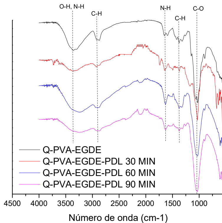
Figura 3.4 Espectro de las esferas de 3.1 mm (sin modificar y modificadas en el reactor con un volumen de 90.3 \text{ cm}^3 ) antes de la sorción.
