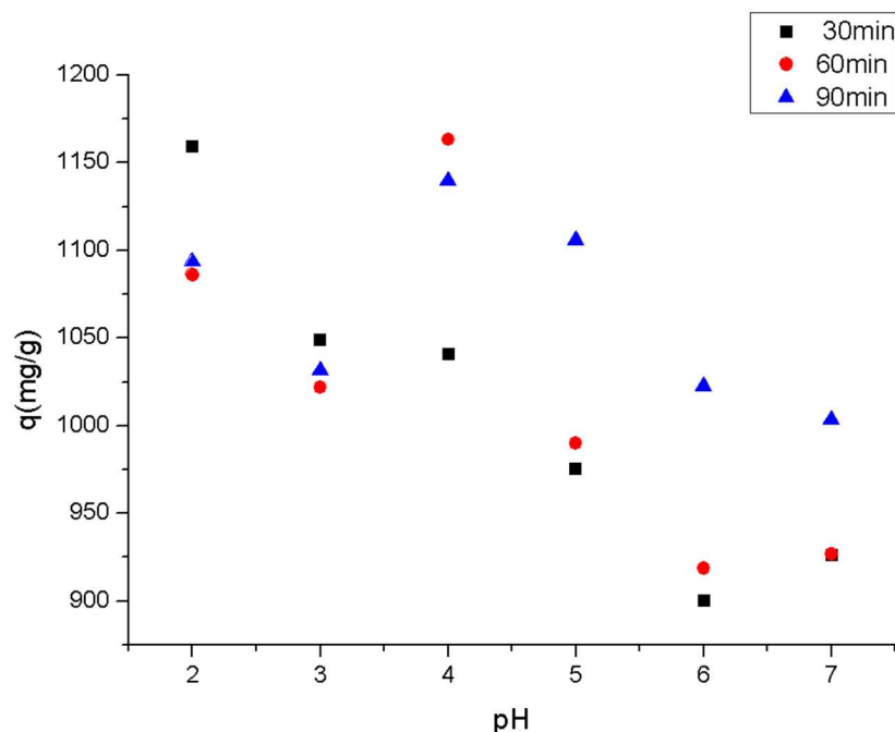
Figura 3.15 Efecto del pH sobre la capacidad de adsorción de la solución con esferas modificadas por plasma a tres diferentes tiempos (esfera de 2.1 mm Ø).
