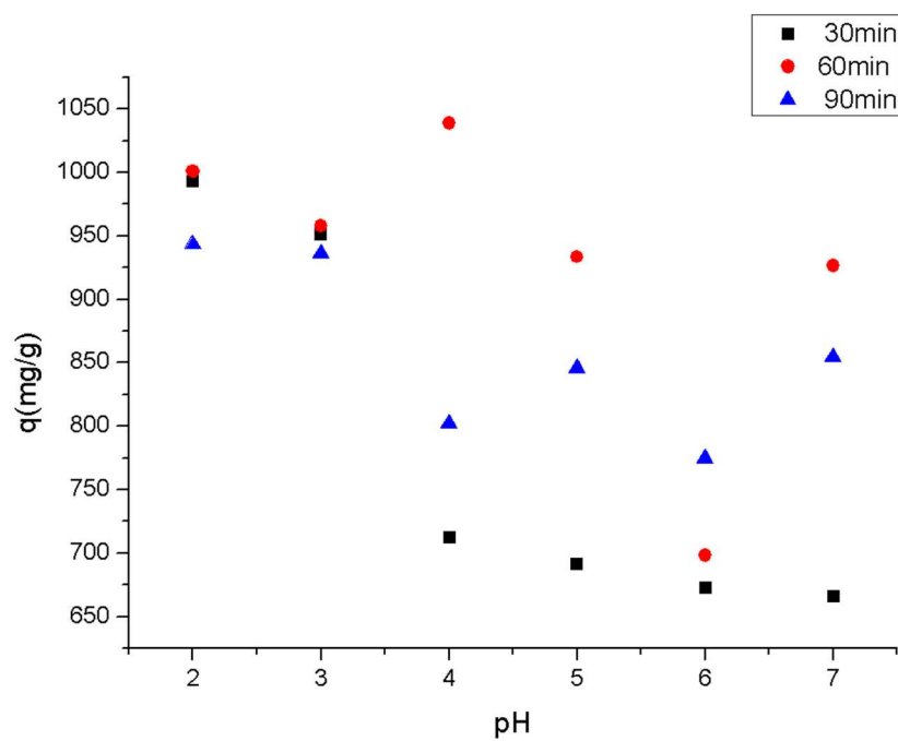
Figura 3.13 Efecto del pH sobre la capacidad de adsorción de la solución con esferas modificadas por plasma a tres diferentes tiempos (esfera de 2.1 mm Ø).
