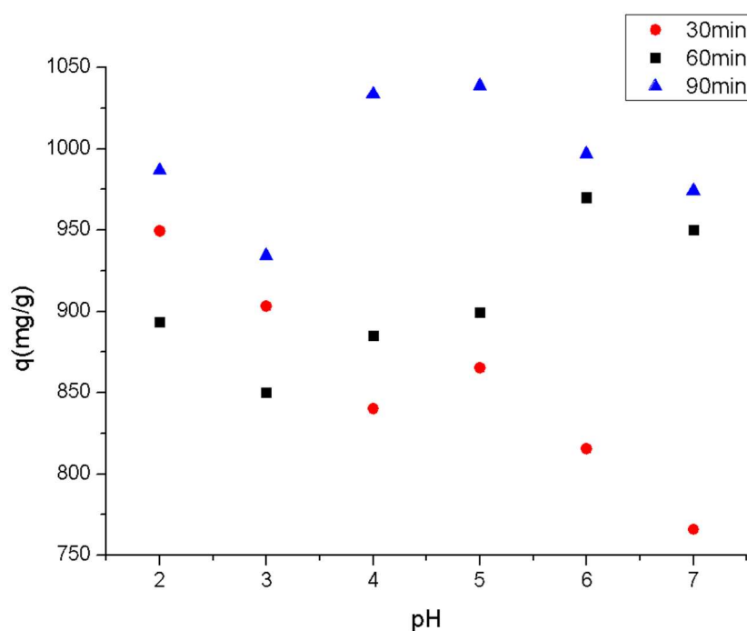
Figura 3.10 Efecto del pH sobre la capacidad de adsorción de la solución con esferas modificadas por plasma a tres diferentes tiempos (esfera de 3.1 mm Ø).
