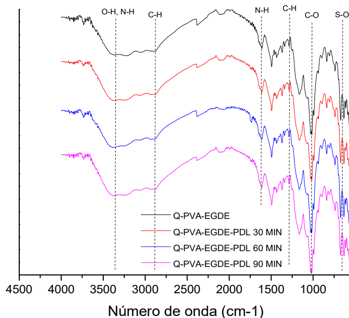
Figura 3.3 Espectros de las esferas de 2.1 mm (sin modificar y modificadas en el reactor con un volumen de 90.3 cm 3 ) después de la sorción.
