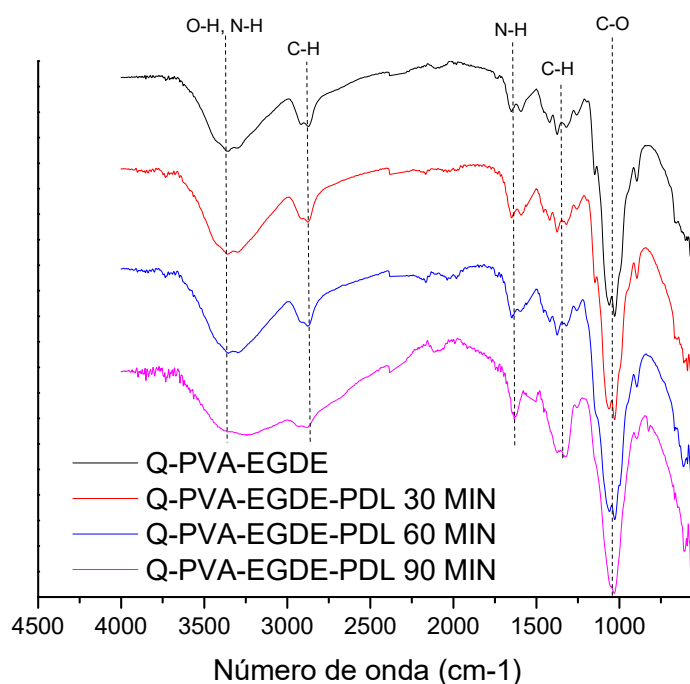
Figura 3.2 Espectros de las esferas de 2.1 mm (sin modificar y modificadas en el reactor con un volumen de 90.3 cm 3 ) antes de la sorción
