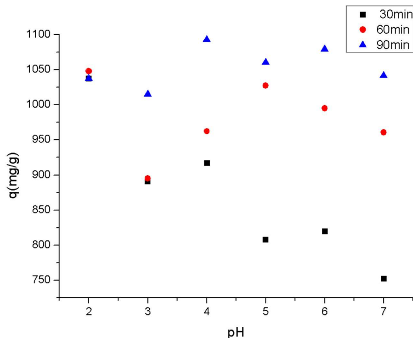
Figura 3.11 Efecto del pH sobre la capacidad de adsorción de la solución con esferas modificadas por plasma a tres diferentes tiempos (esfera de 2.1 mm Ø).
