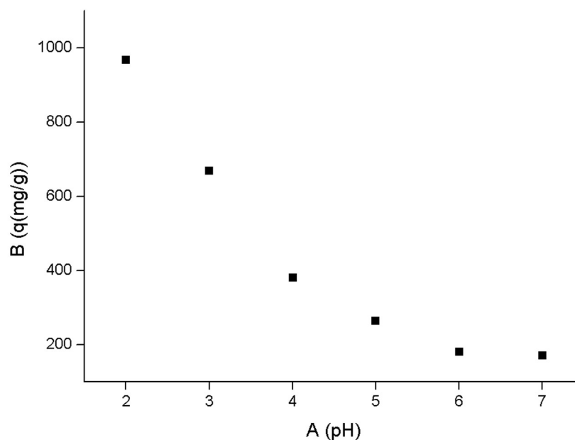
Figura 3.8 Efecto del pH de la solución inicial para esfera de 3.1 mm.
