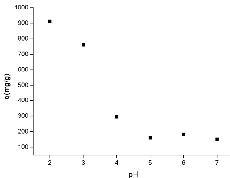
Figura 3.9 Efecto del pH de la solución para esfera de 2.1 mm.
