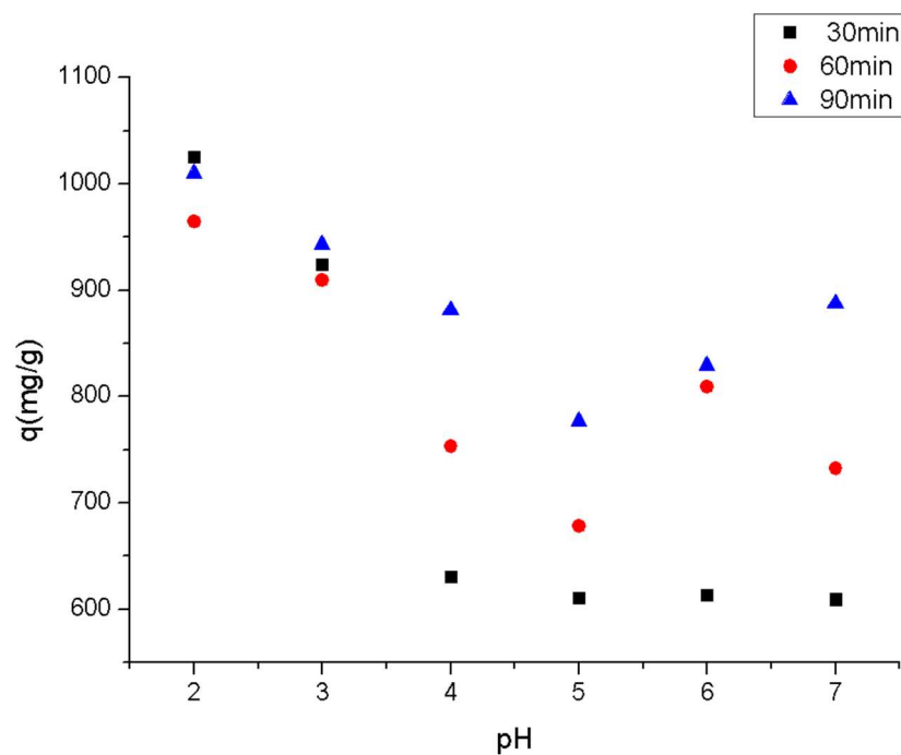
Figura 3.12 Efecto del pH sobre la capacidad de adsorción de la solución con esferas modificadas por plasma a tres diferentes tiempos (esfera de 3.1 mm Ø).
