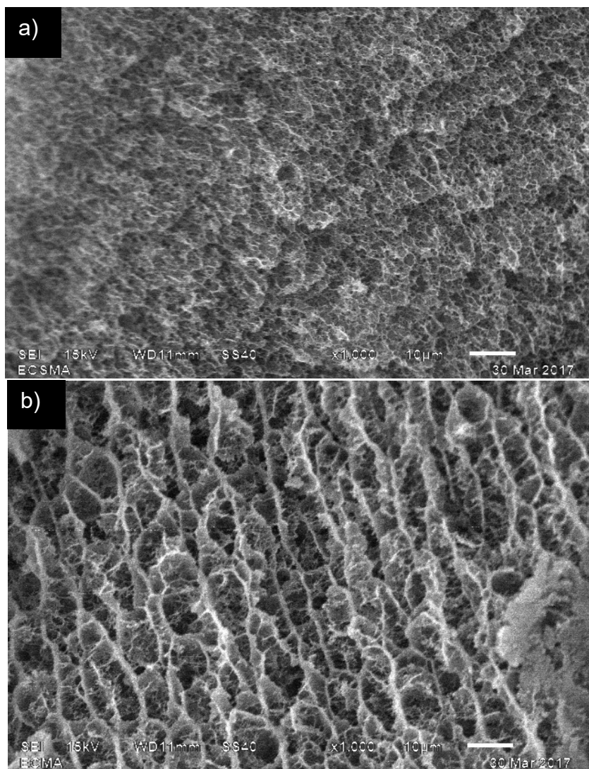
Figura 3.7 Micrografías de las esferas Q-PVA-EGDE a) Esferas sin modificar b) Esferas modificadas por PDL.
