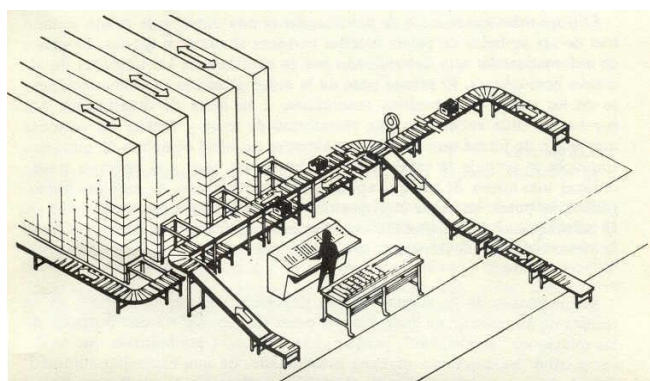
Figuras 4.21 y 4.22 Manejo manual, mecanizado y automatizado
