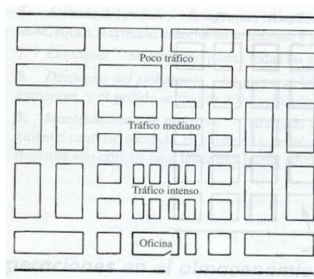
Figura 4.12 Distribución por frecuencia de movimientos.
