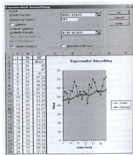
Figura 2.10: Aplicación del método de suavización exponencial.
