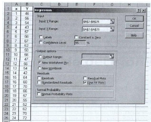
Figura 2.11: Aplicación de regresión Excel
