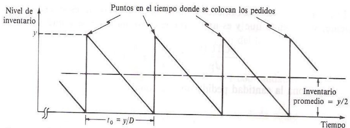
Figura 3.6 Comportamiento del inventario en el modelo CEP o EOQ clásico
