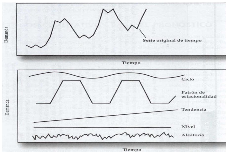
Figura 2.3: Series de tiempo
