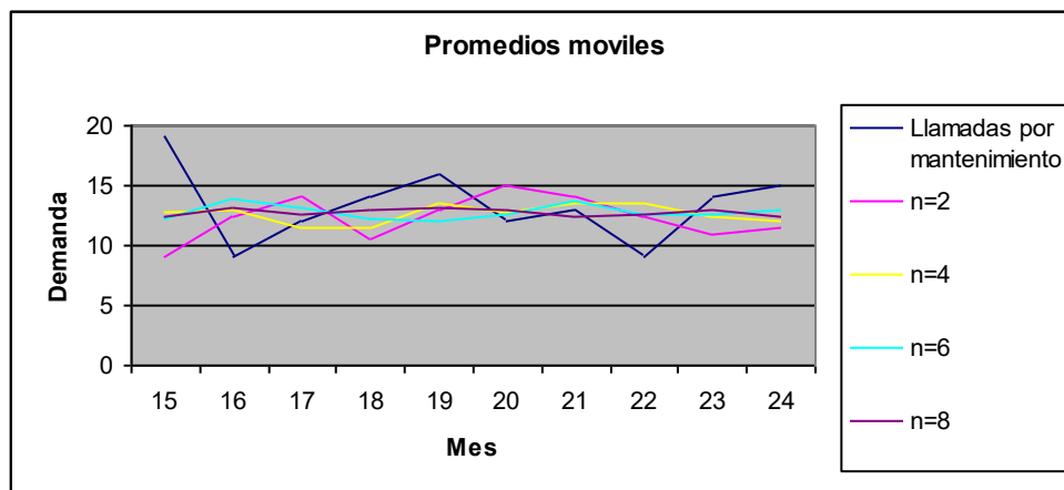
Figura 2.4: Gráfica de promedios móviles
