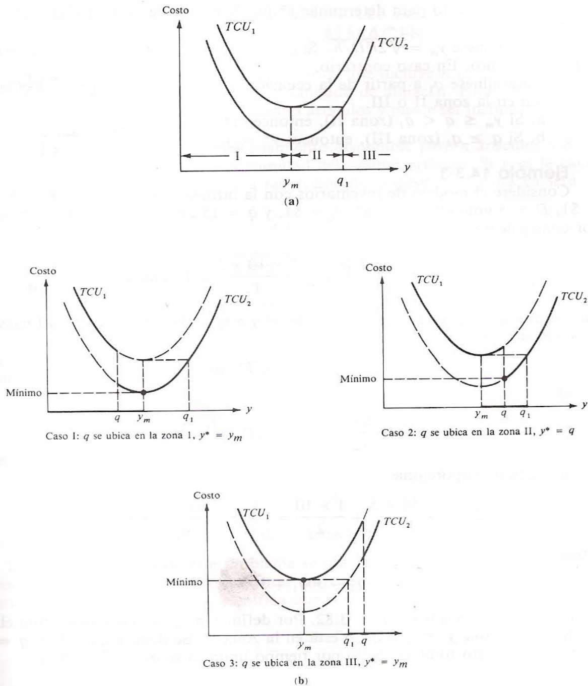
Figura 3.8 Función de costo y solución óptima de inventario con descuento.
