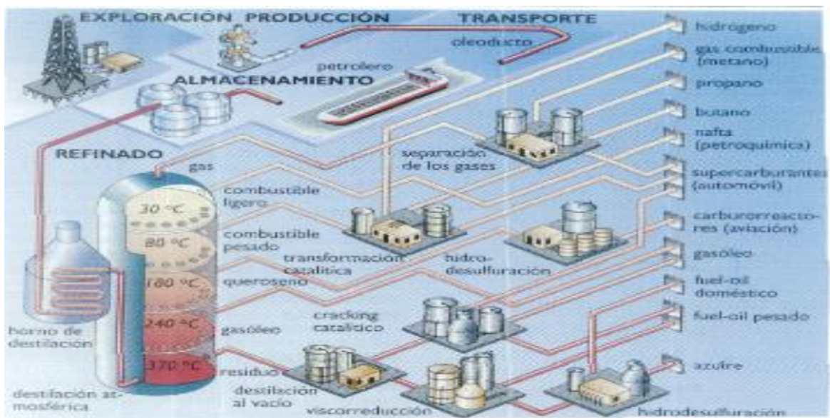
FIGURA 1.6: El ciclo del petróleo desde la explotación hasta la extracción y refinado.
