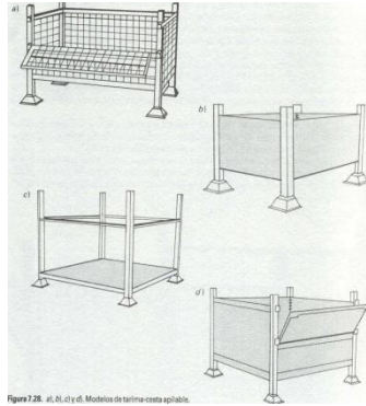
Figura 4.24 Modelos de tarima/cesta apilable.
