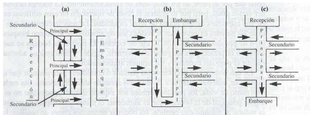
Figura 4.9 Configuración de pasillos
