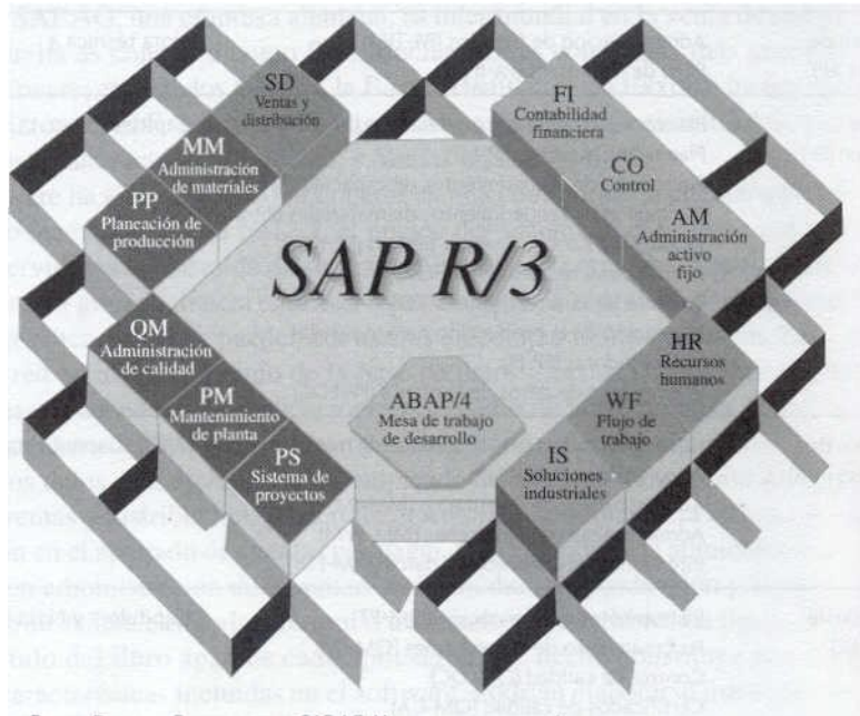
Figura 4.30 Módulos de aplicaciones del R/3.
