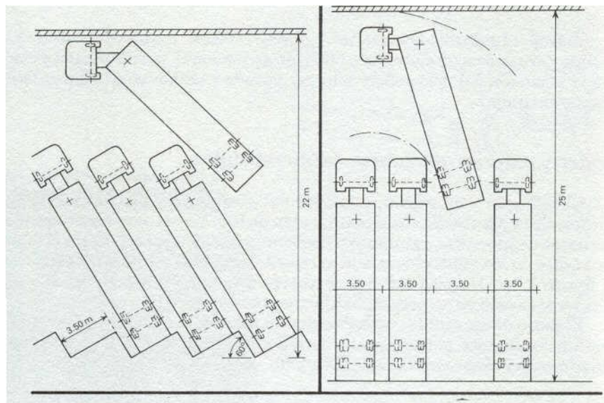
Figura 4.4 patio de maniobras de los vehículos.
