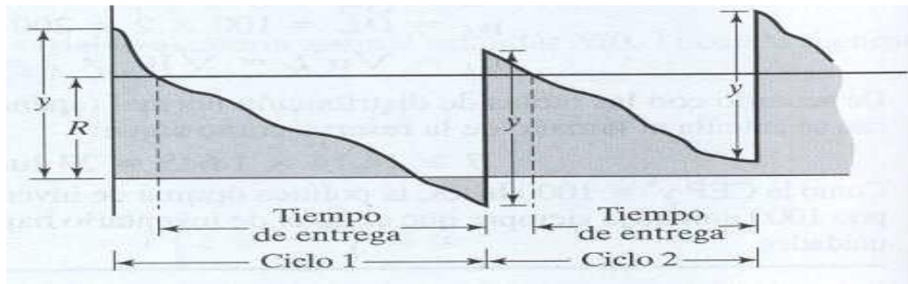
Figura 3.11 Modelo probabilístico de inventario
