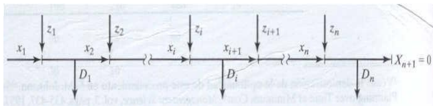
Figura 3.9 Elementos de modelo del modelo dinámico de inventario.
