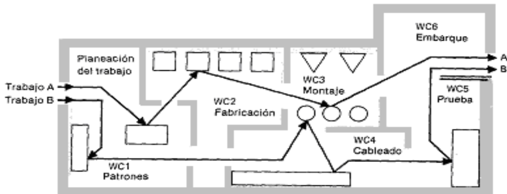
Figura Distribución por proceso para la producción de señales
