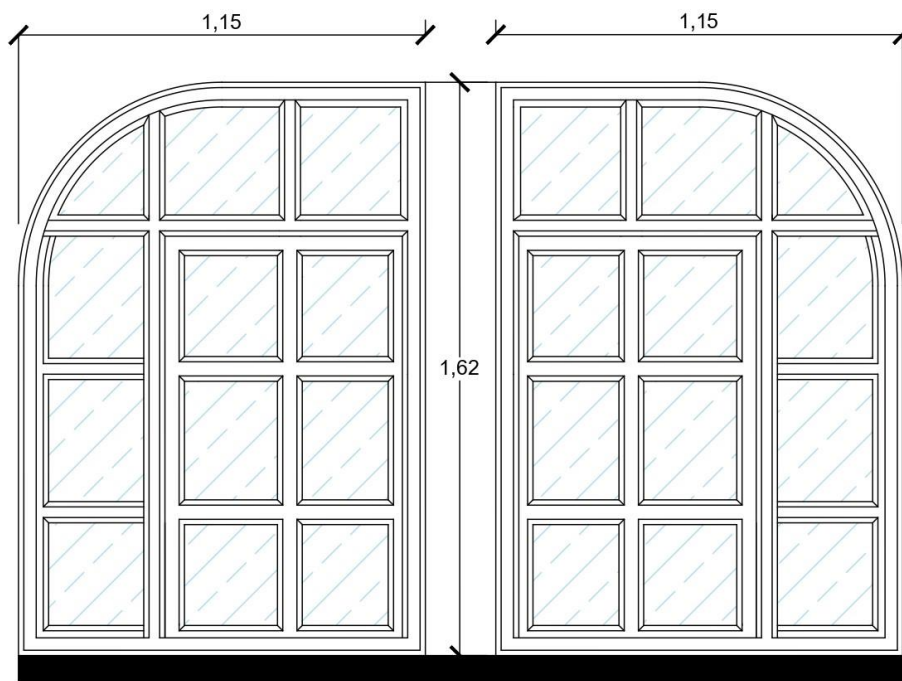
Ventana de madera con medio arco rebajado V2-00A1
