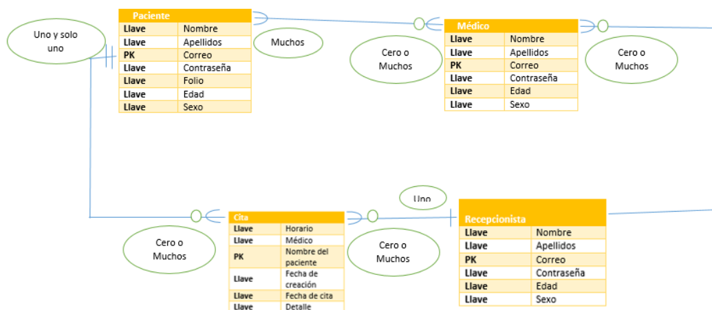
Ilustración 75 Modelo entidad-relación
