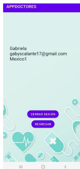
Ilustración 98 Perfil administradora
