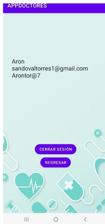
Ilustración 103 Perfil médico
