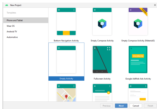
Ilustración 9 Empty Activity
