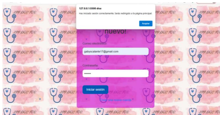
Ilustración 104 Iniciar sesión
