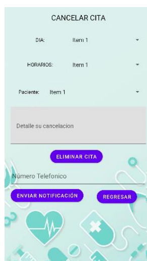
Ilustración 66 Cancelar cita
