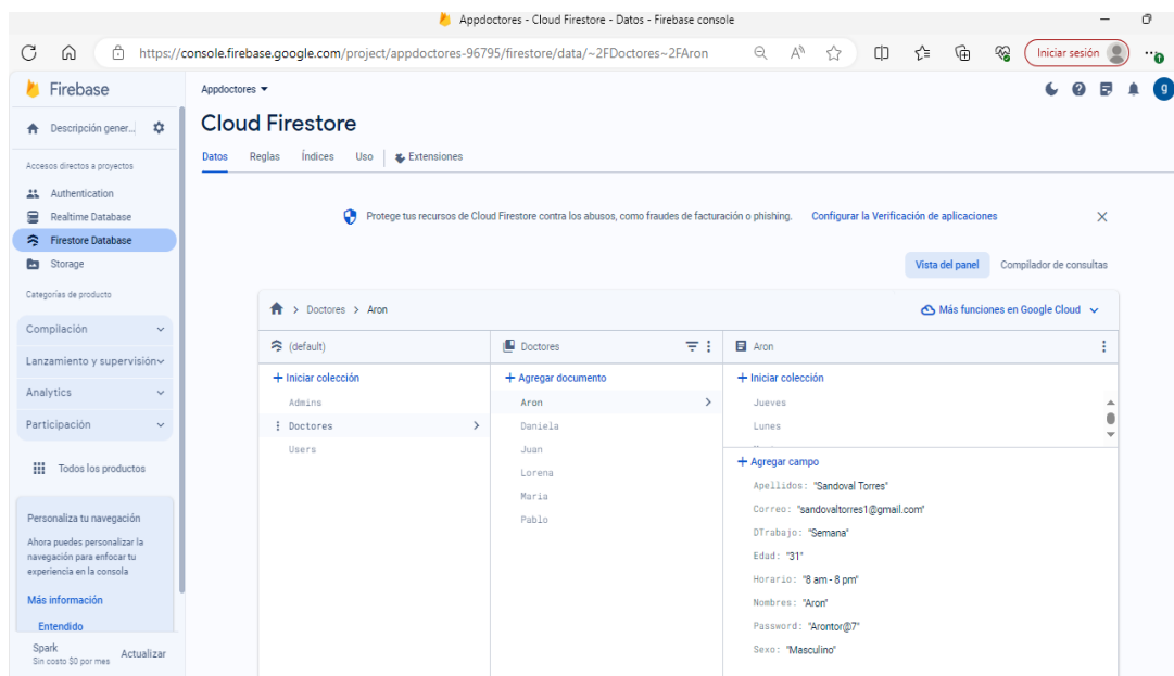
Ilustración 108 Colecciones
