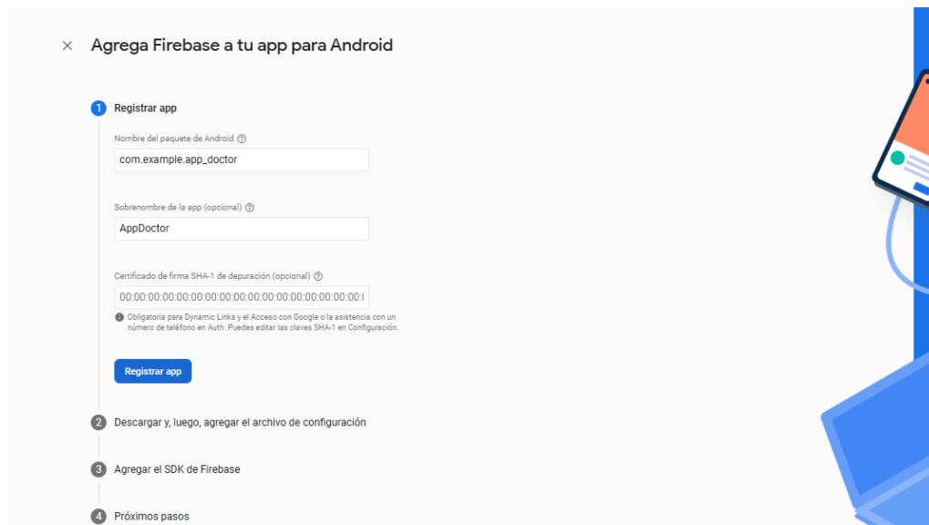
Ilustración 17 Registrar app
