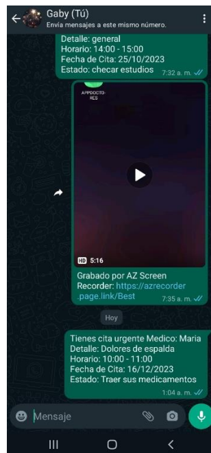
Ilustración 97 Avisar médico
