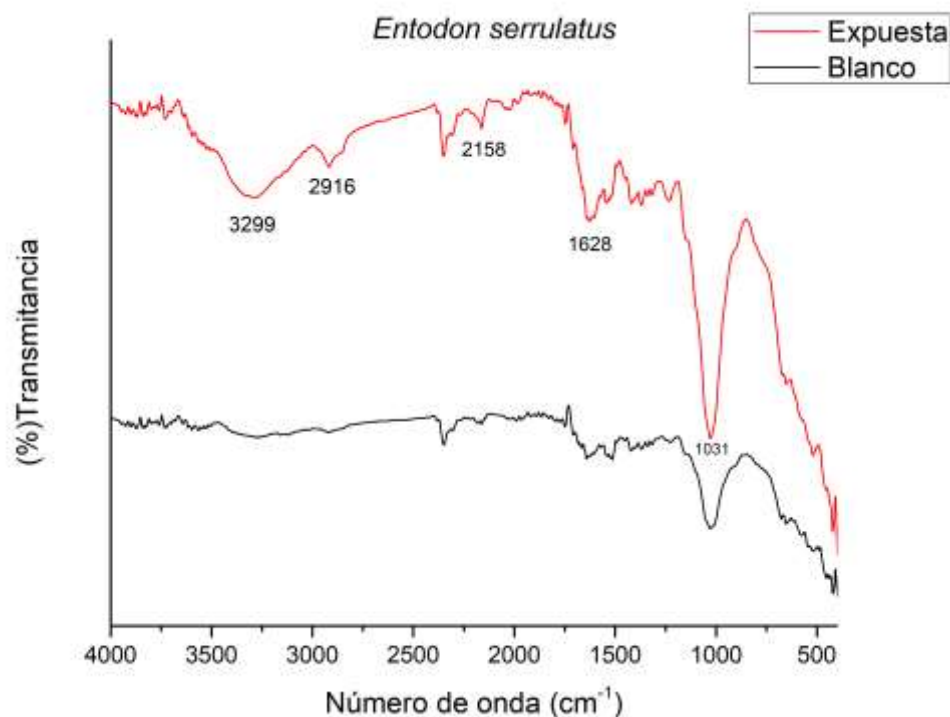
Figura 17 FTIR de Entodon serrulatus antes y después de la exposición
