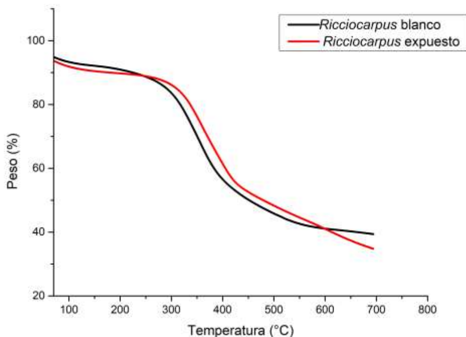
Figura 18 TGA de Ricciocarpus natans antes y después de 6 meses de exposición
