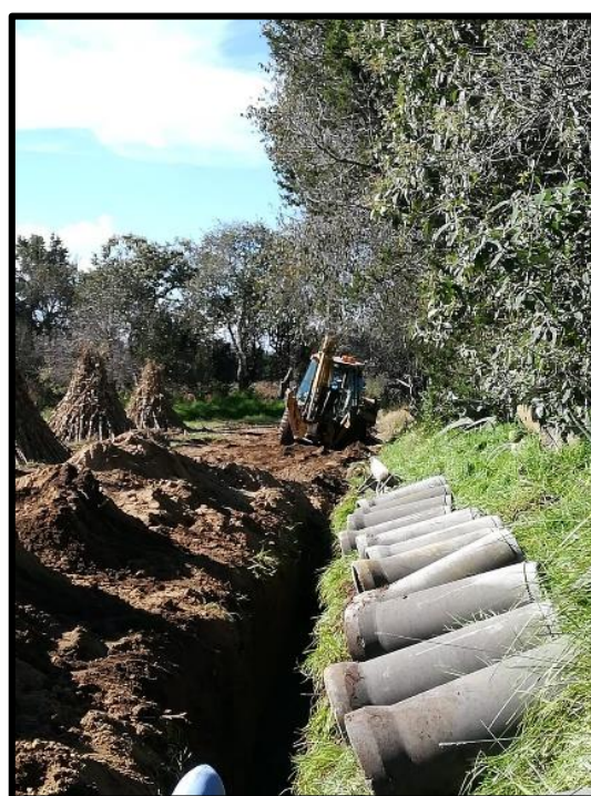
IMAGEN 12 TENDIDO DE TUBERÍA DE CONCRETO SIMPLE CON UN DIÁMETRO DE 18 PULGADAS.
