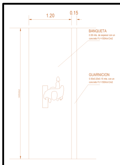
DETALLES DE CONSTRUCCIÓN DE GUARNICIONES Y BANQUETAS
