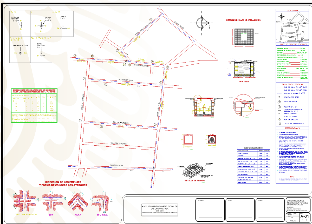
PLANOS 1 RED DE DISTRIBUCIÓN DE LÍNEA DE AGUA POTABLE
