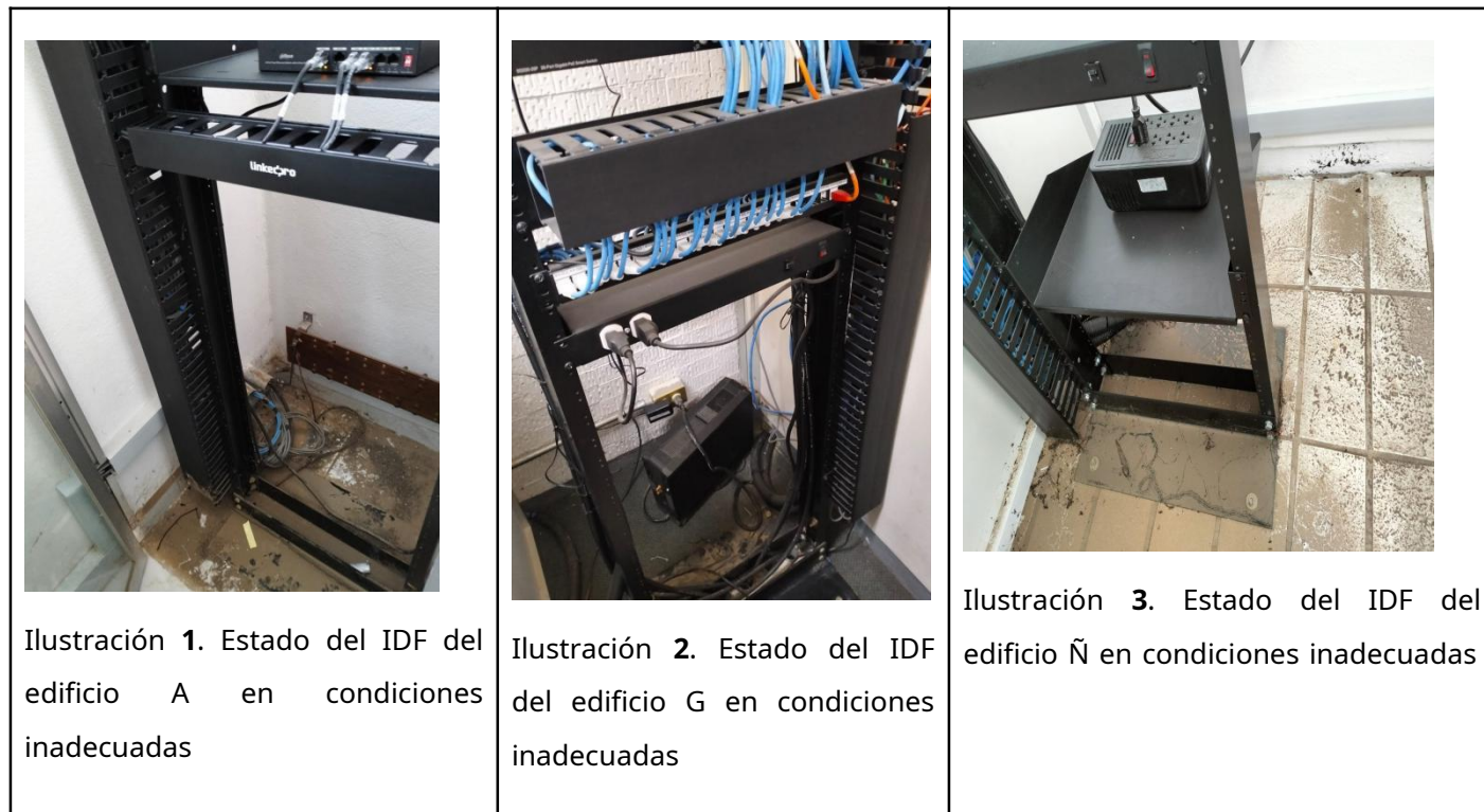
Figura 4 Evidencia del estado físico deteriorado de los racks de comunicaciones.
