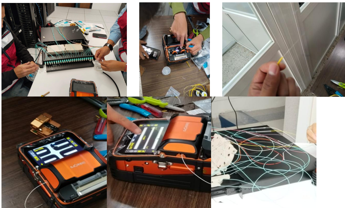
Figura 11 Proceso de fusión de fibra óptica.
