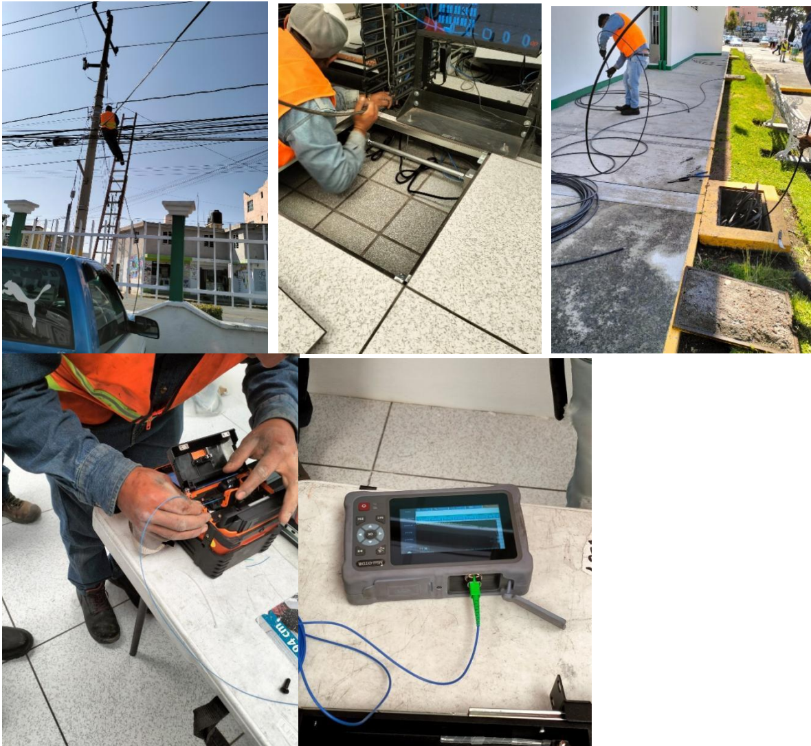
Figura 19 Supervisión del tendido y fusión de fibra óptica hacia el Edificio R (MDF)
