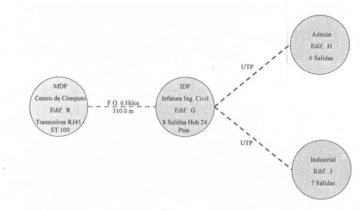
Figura 1 Enlaces troncales de la red del ITA: primeras conexiones hacia la mitad del campus.
