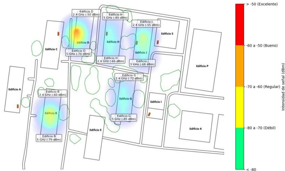
Figura 29 Mapa de calor de cobertura inalámbrica con puntos de acceso instalados
