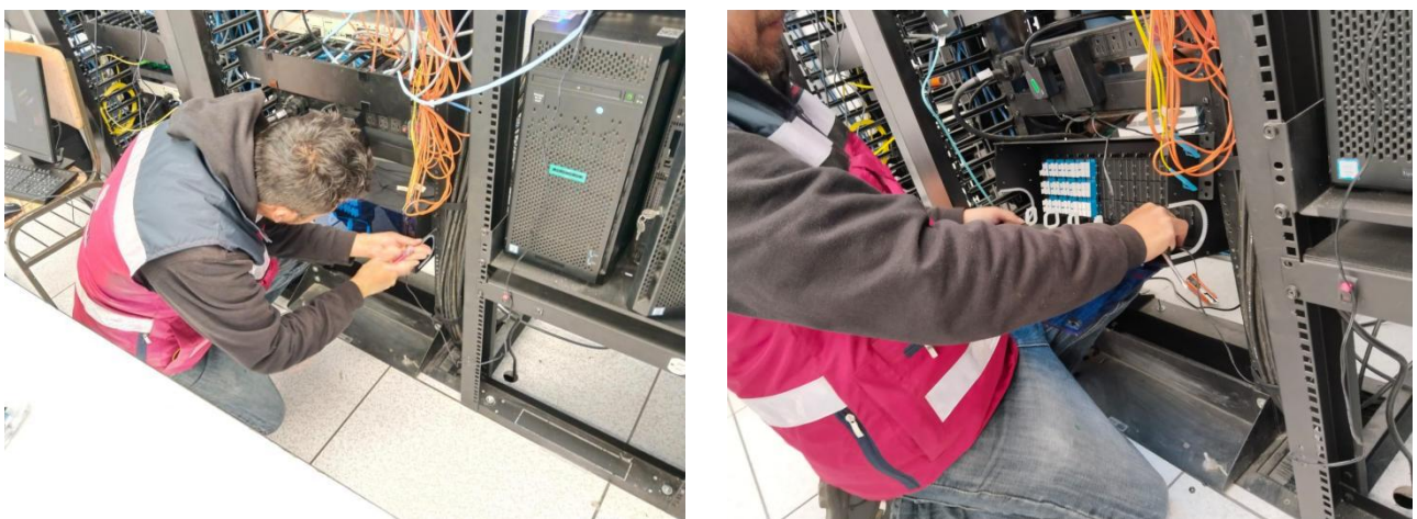
Figura 7 Tendido de cable de fibra óptica como parte del backbone de red institucional.
