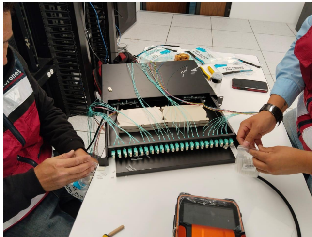
Figura 23 Gabinete para fibra óptica y fusionadora.
