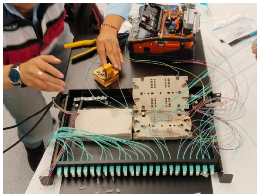
Figura 18 Montaje de la infraestructura cableada de fibra óptica.
