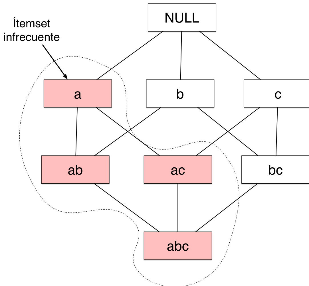
Figura 60: Rejilla de ítemset
