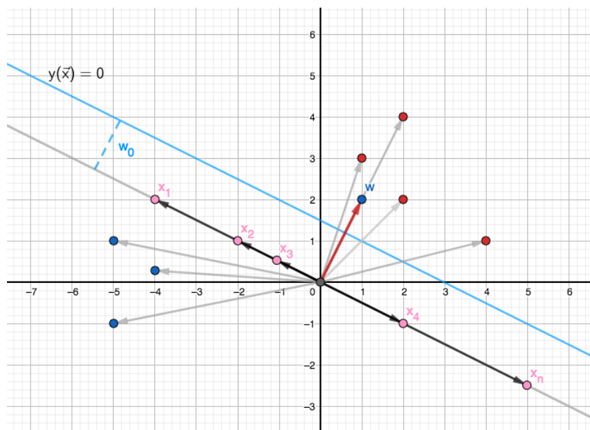
Figura 52: Función discriminante definida por \vec{w} , vectores ortogonales más un sesgo w_0 , en azul
