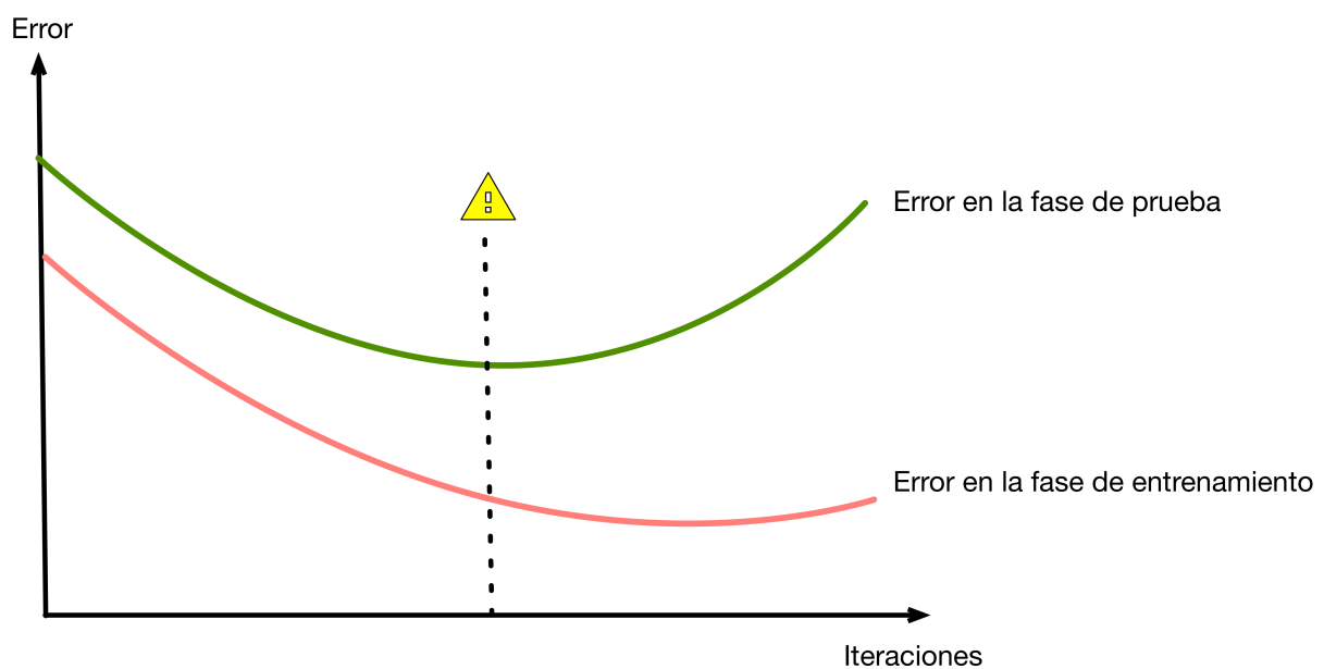
Figura 48: Relación entre la cantidad de entrenamiento y los errores en las etapas de prueba y entrenamiento
