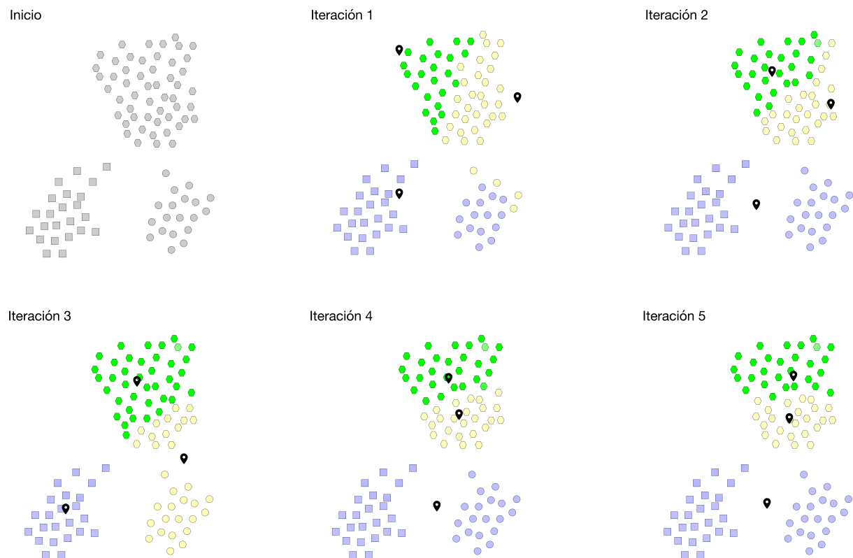
Figura 67: Incorrecta selección de posiciones iniciales de los centroides
