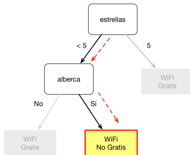
Figura 44: Ruta de disparo para clasificar el registro de prueba
