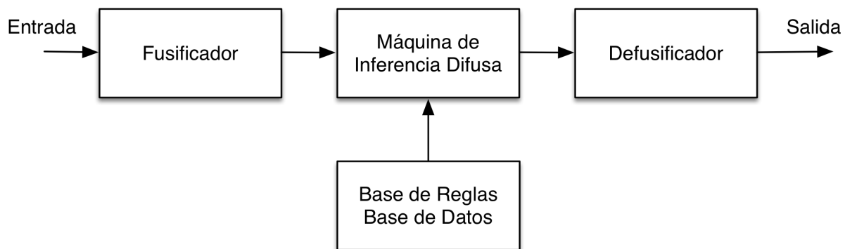
Figura 41: Componentes Principales de un Sistema de Inferencia Difuso
