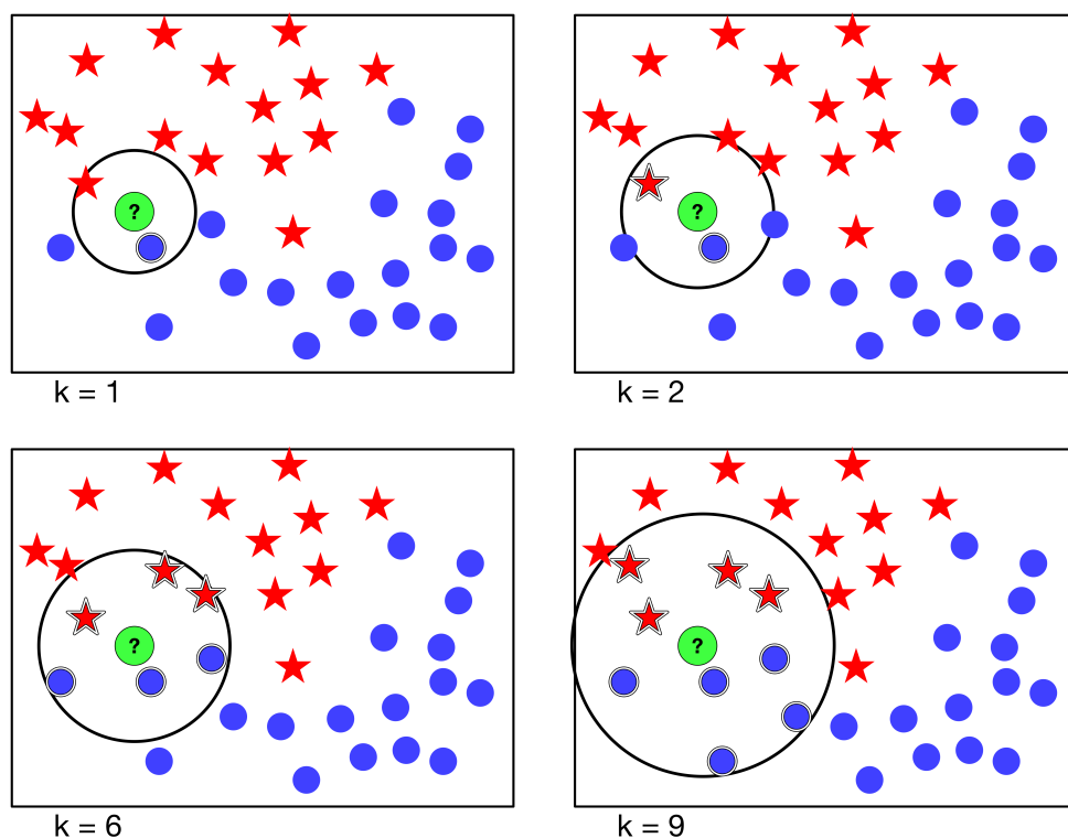
Figura 49: Efecto de la elección del número de vecinos k
