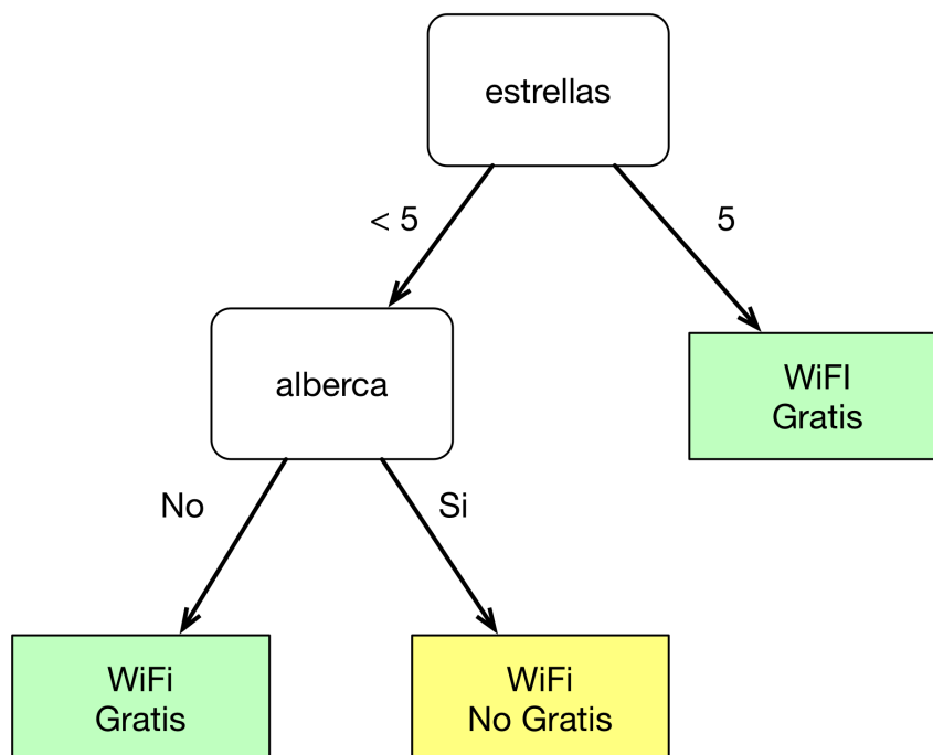
Figura 43: Árbol de decisión propuesto
