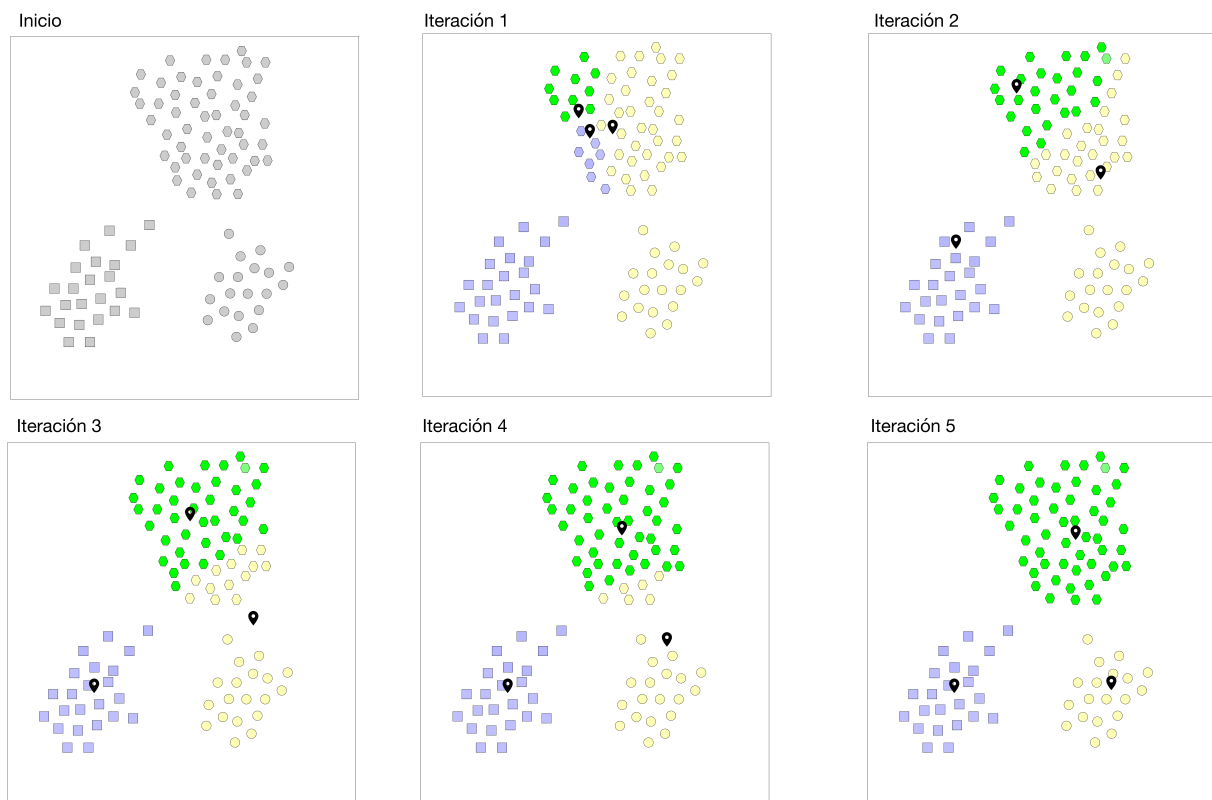
Figura 66: Ejemplo del algoritmo k -medias
