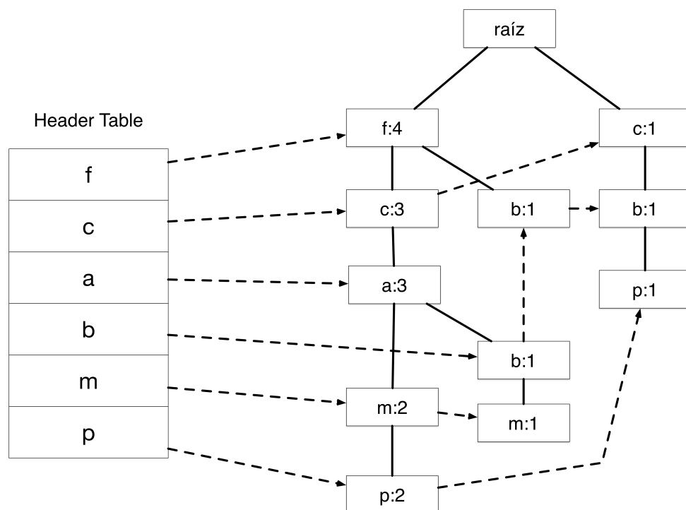
Figura 62: Ejemplo de F-Tree Han, Pei, and Yin (2000)
