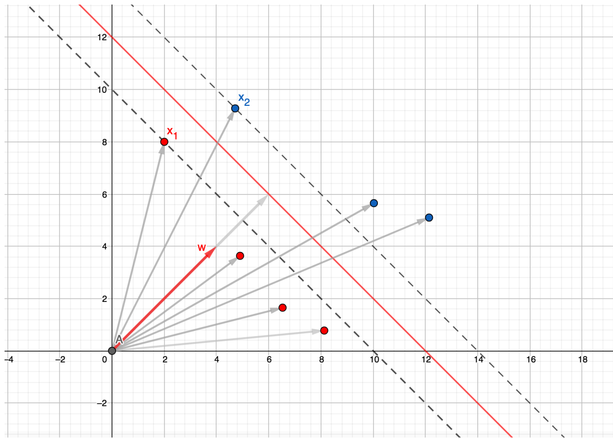
Figura 56: Vectores de soporte
