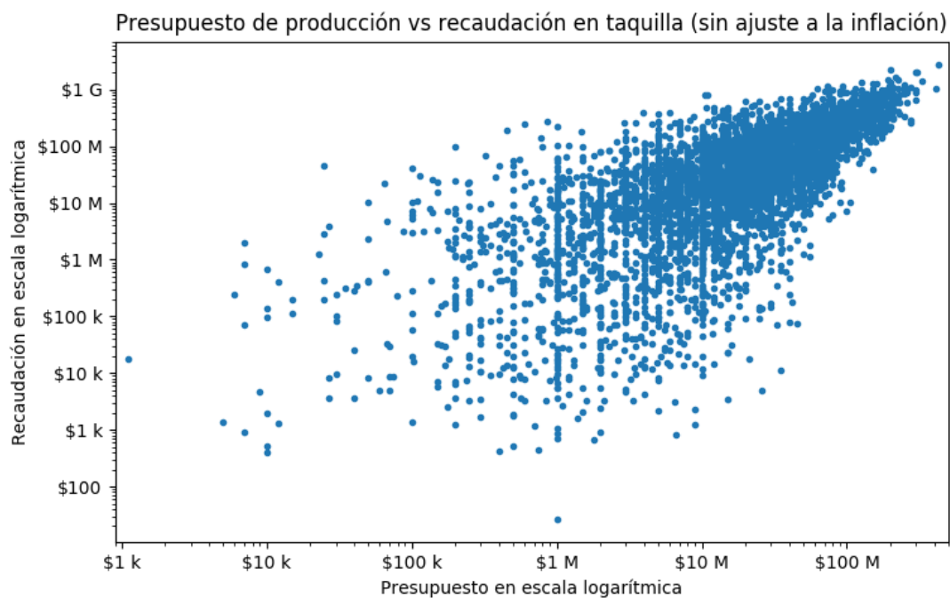
Figura 28: Presupuesto vs recaudación escala logarítmica
