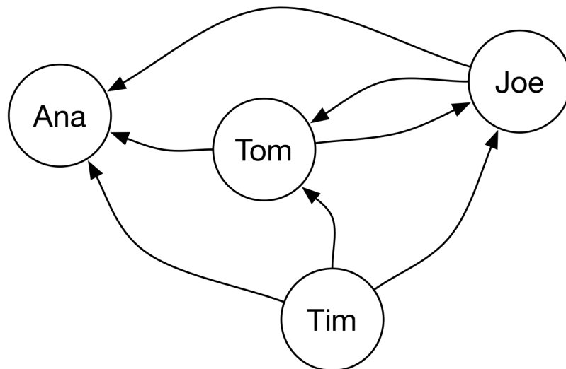
Figura 9: Una matriz expresada en forma de grafo
