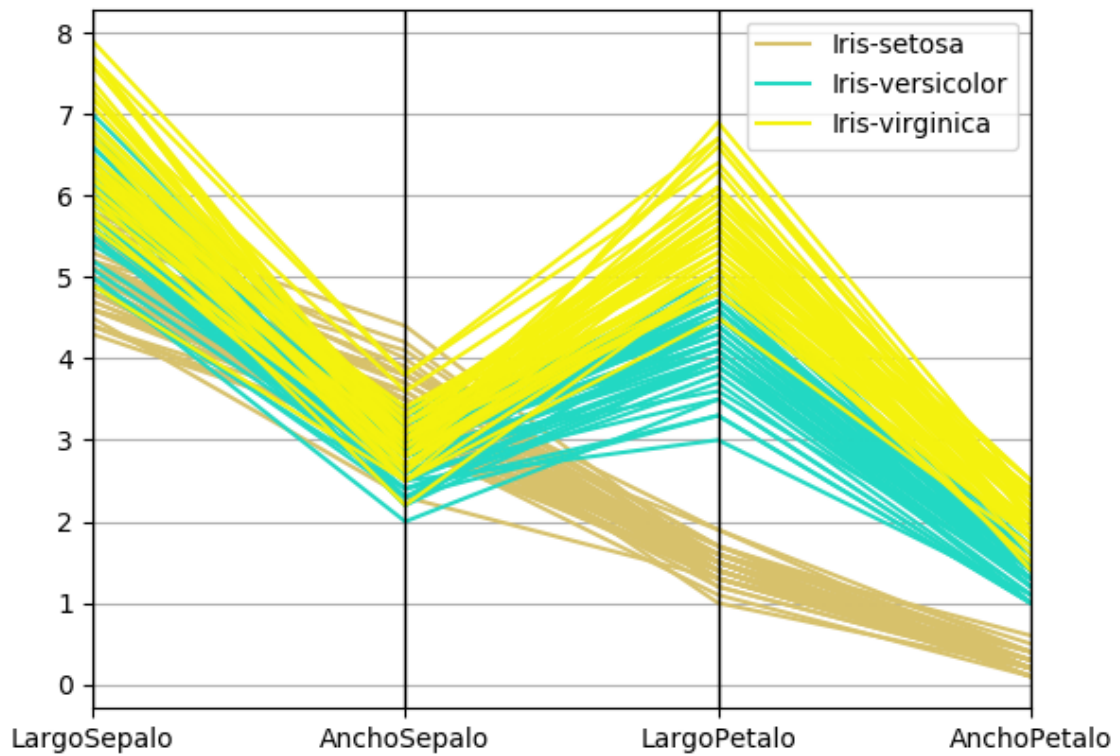
Figura 36: Gráficas paralelas que representan las cuatro variables del conjunto de datos Iris
