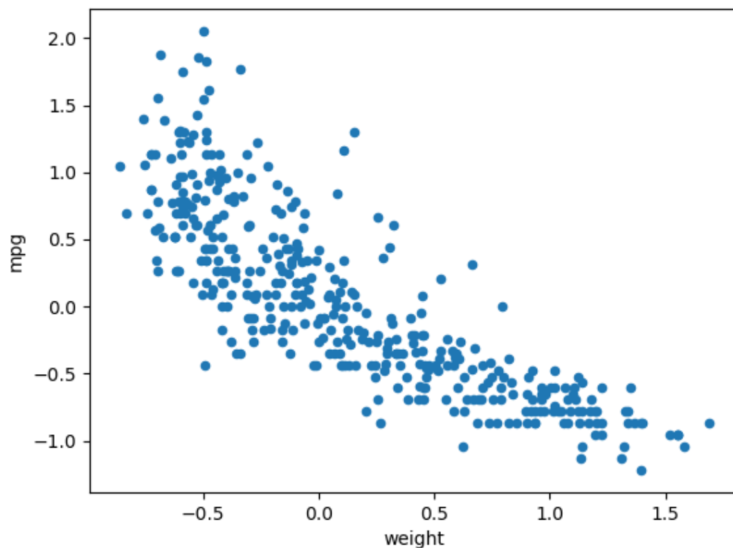
Figura 18: MPG Data
