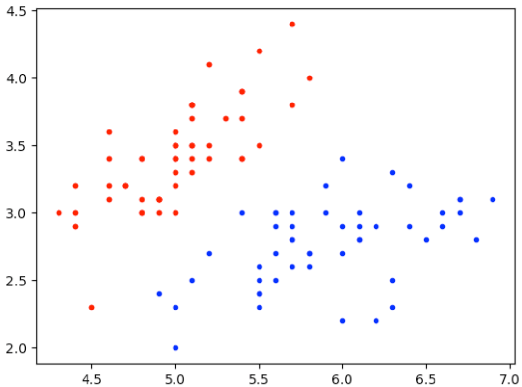
Figura 4: Setosa y Virginica
