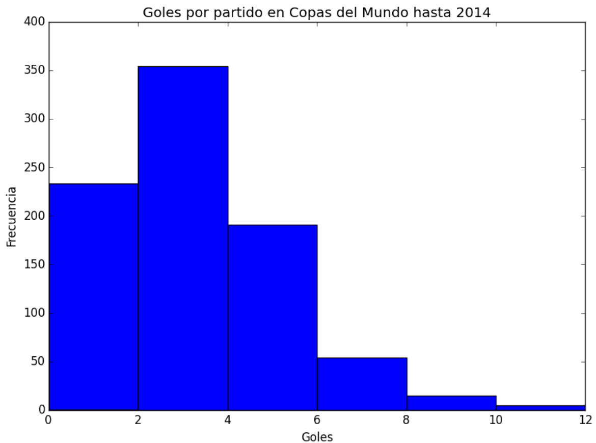
Figura 30: Goles por partido en Copas del Mundo
