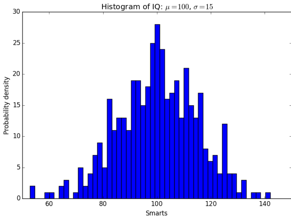
Figura 31: Histograma de datos continuos
