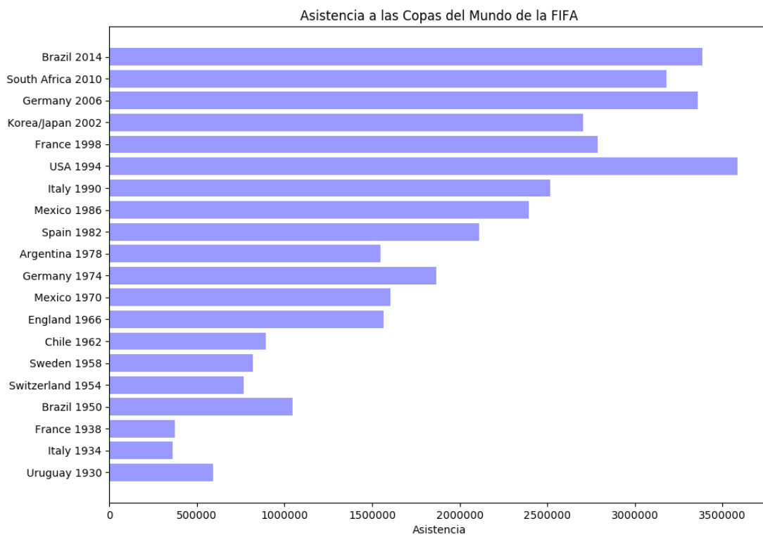
Figura 29: Asistencia a las Copas del Mundo de la FIFA
