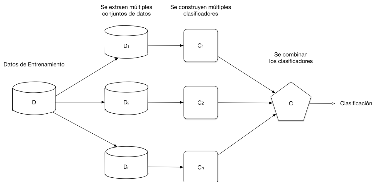
Figura 57: Esquema general del aprendizaje ensemble
