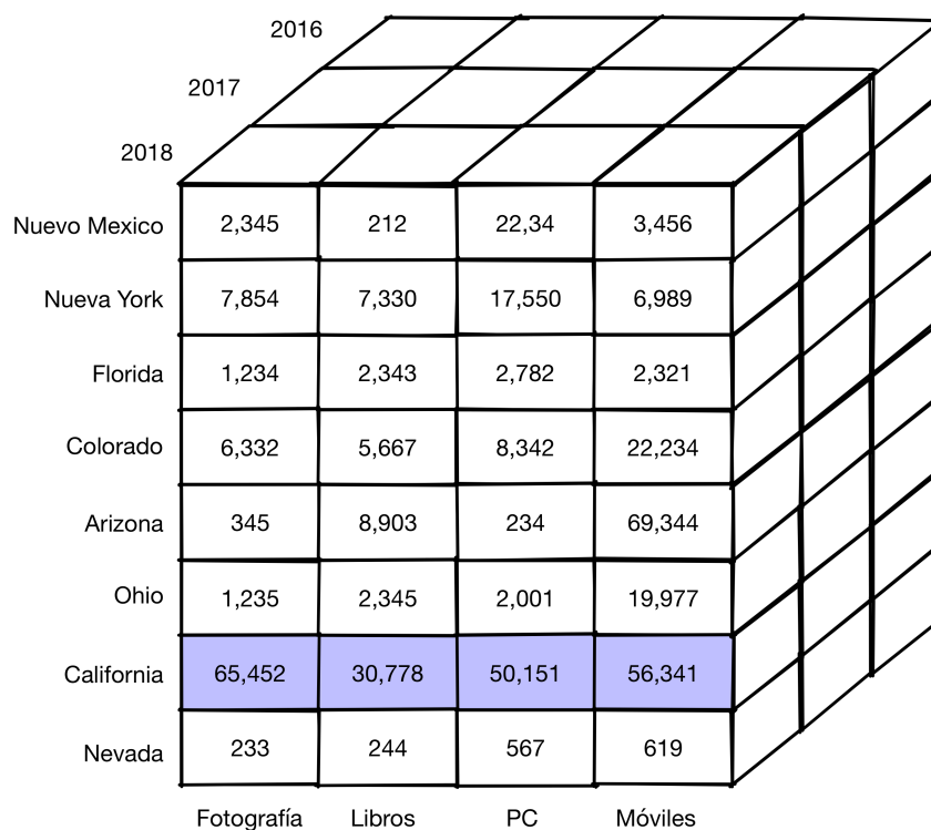
Figura 39: Cubo OLAP para el almacén de ventas
