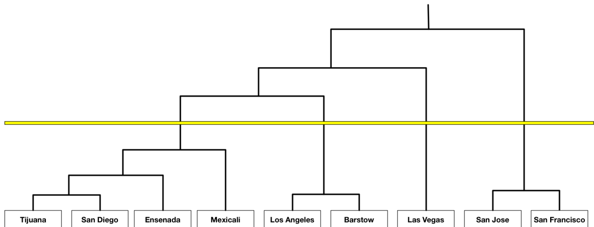
Figura 71: Ejemplo de agrupamiento jerárquico
