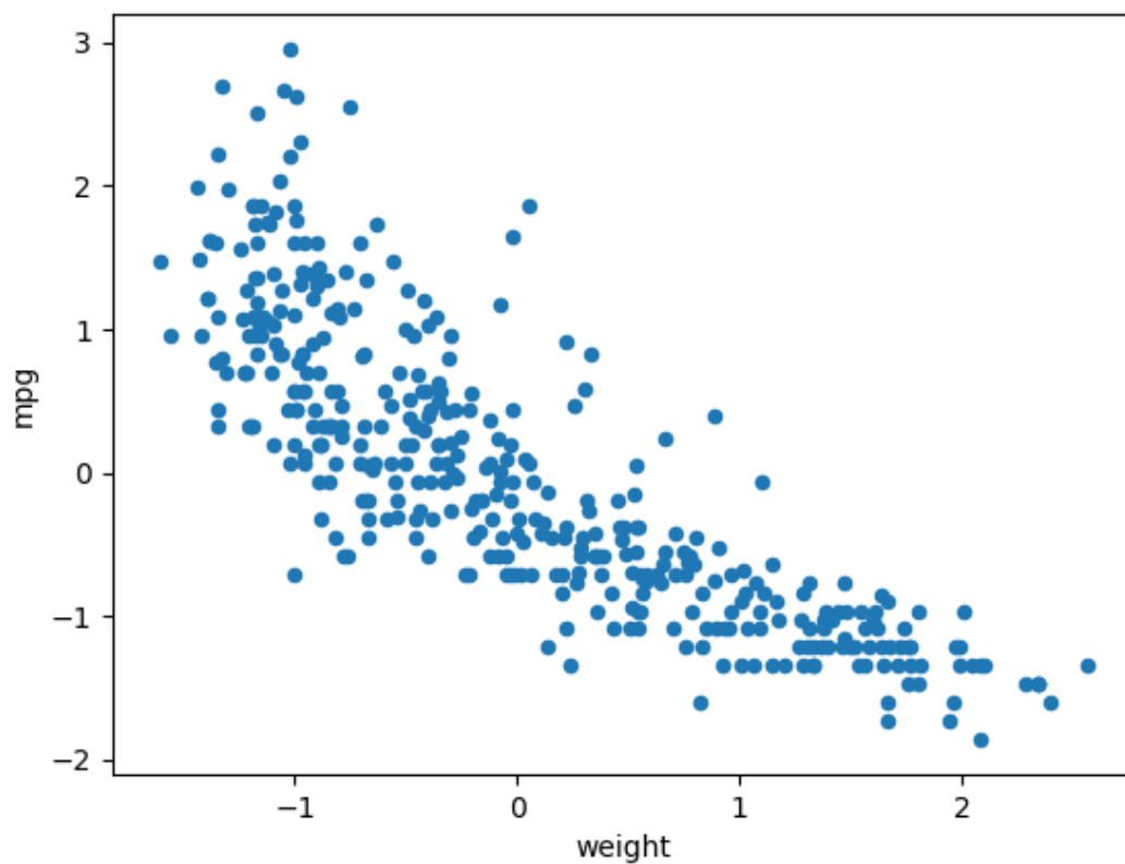
Figura 15: MPG Data
