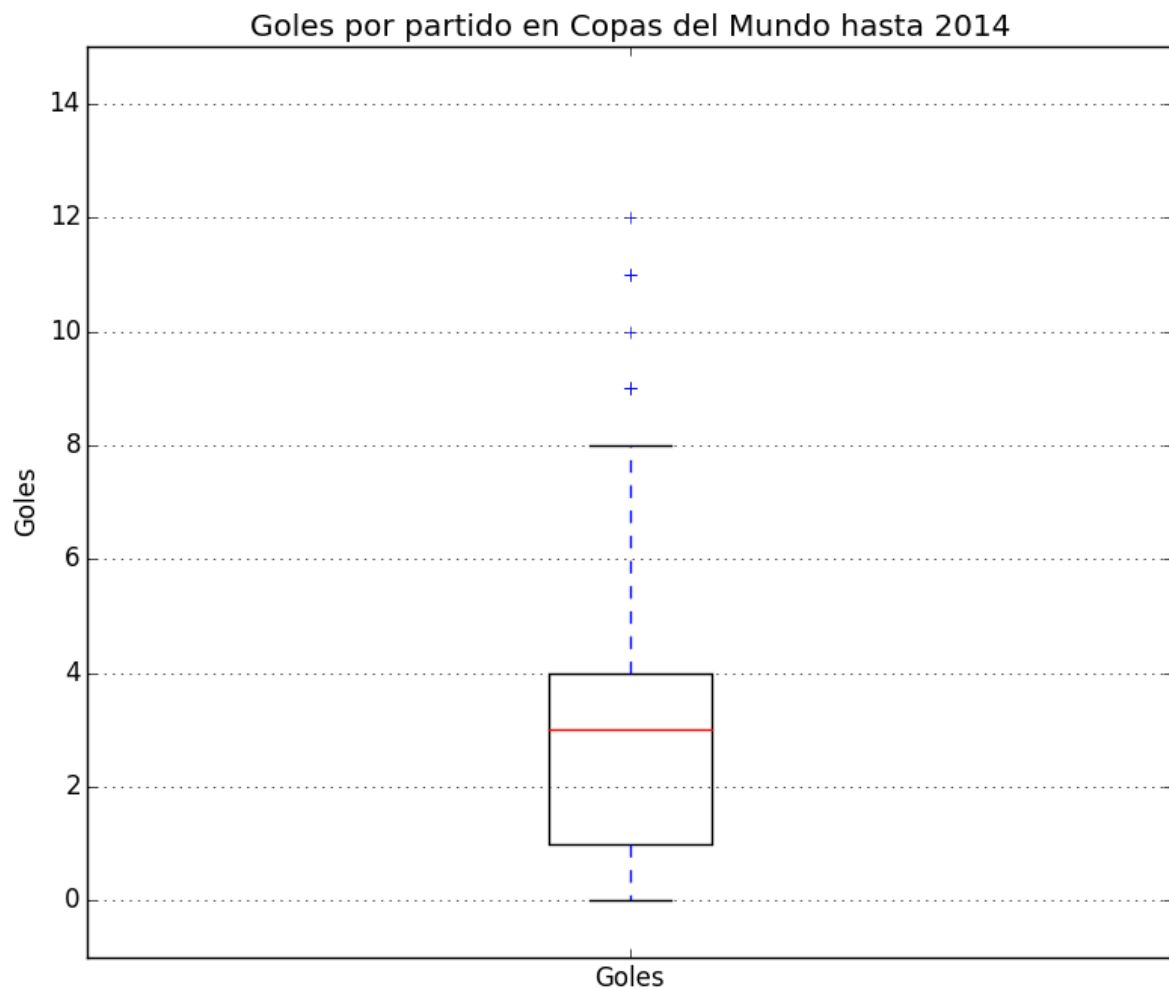
Figura 33: Goles por partido en Copas del Mundo
