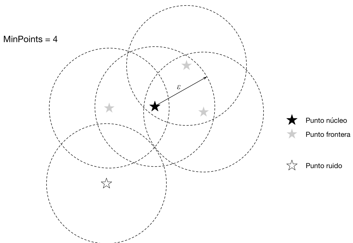
Figura 73: Agrupación DBSCAN
