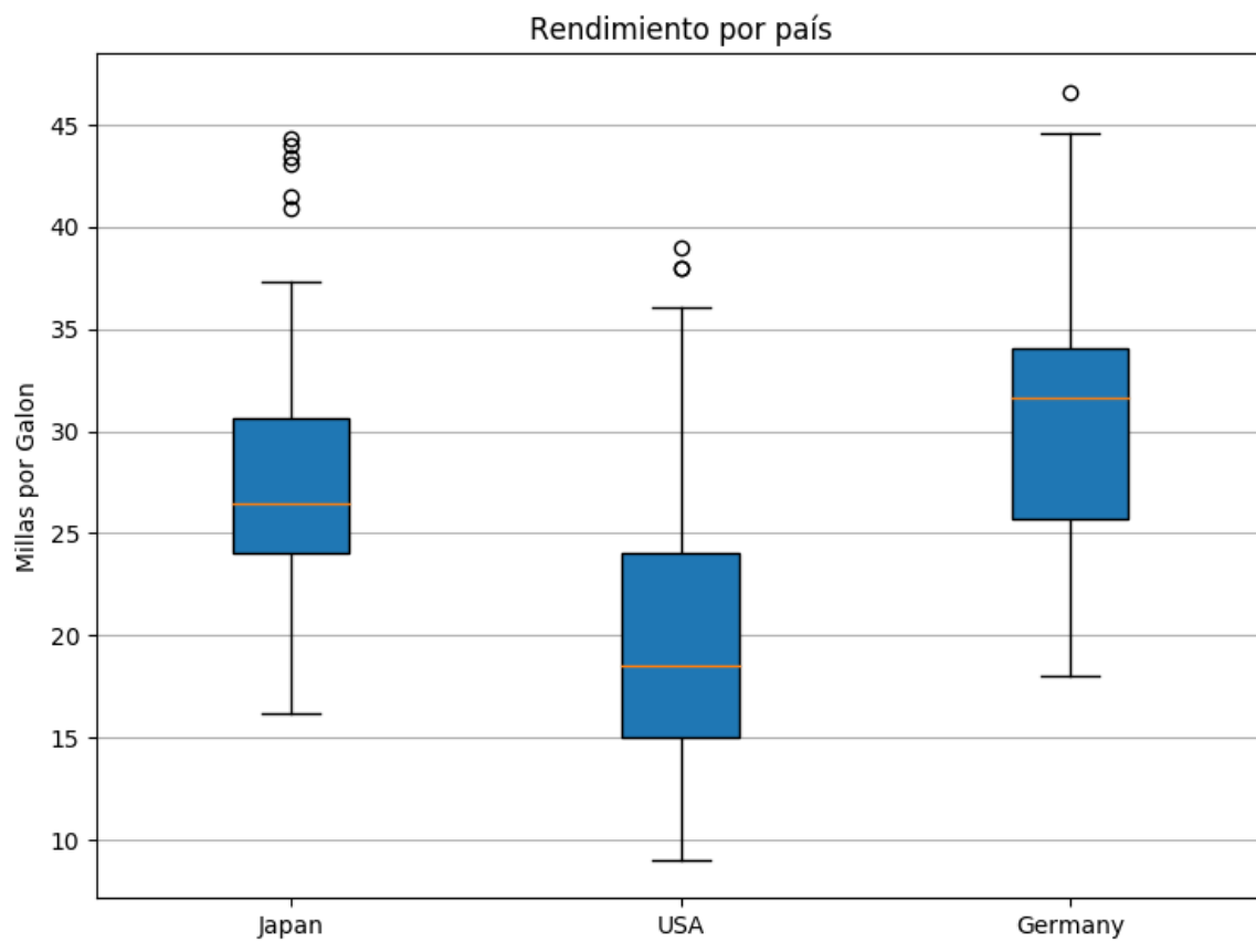
Figura 34: Diagrama de Cajas del rendimiento en MPG de los autos fabricados por Japón, Estados Unidos y Alemania.
