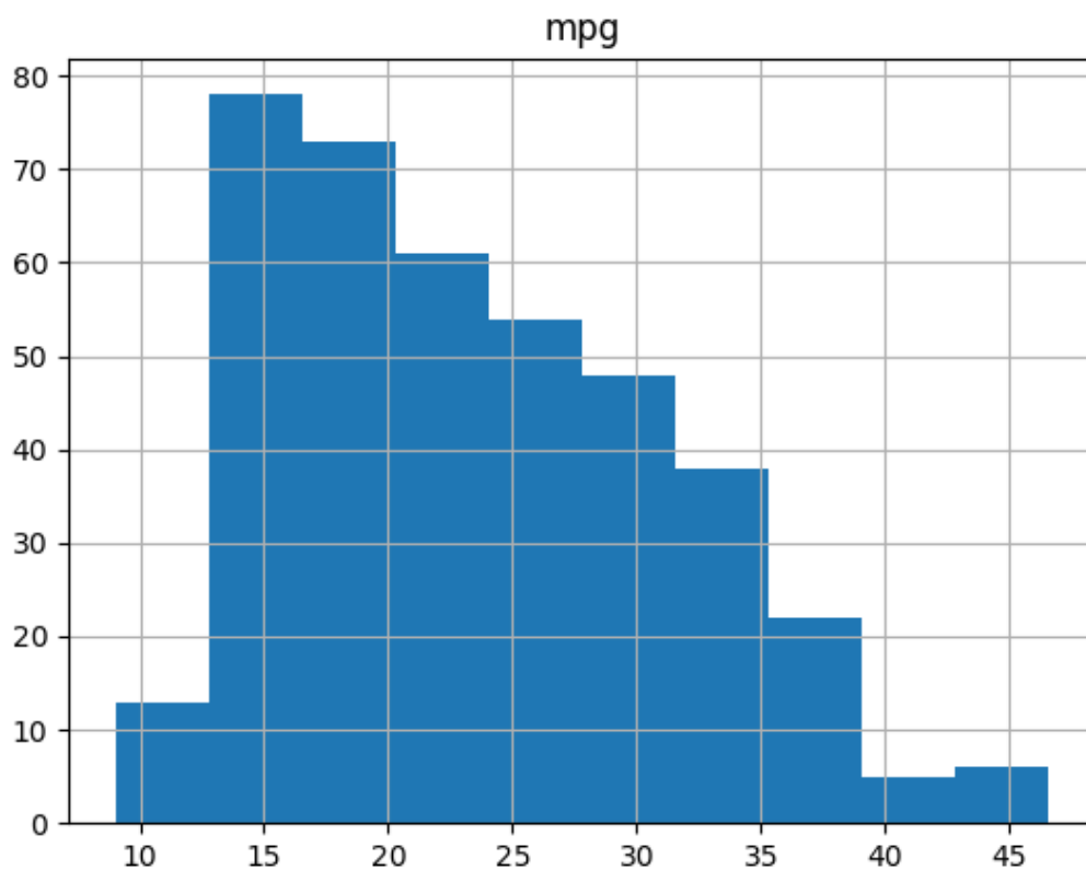
Figura 13: MPG Data
