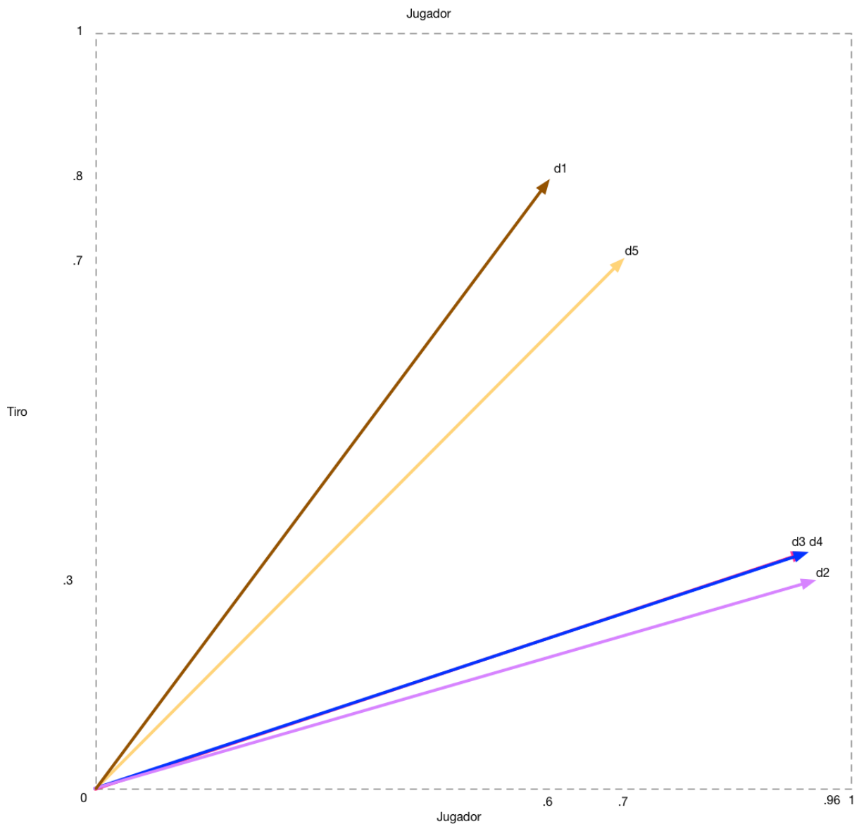
Figura 20: Norma L_2
