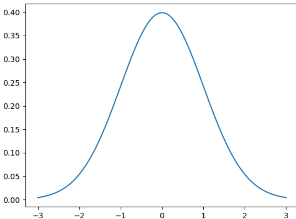
Figura 14: estandar
