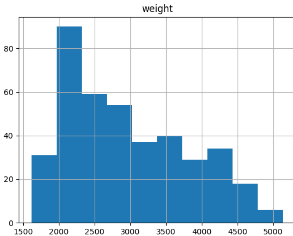
Figura 12: MPG Data
