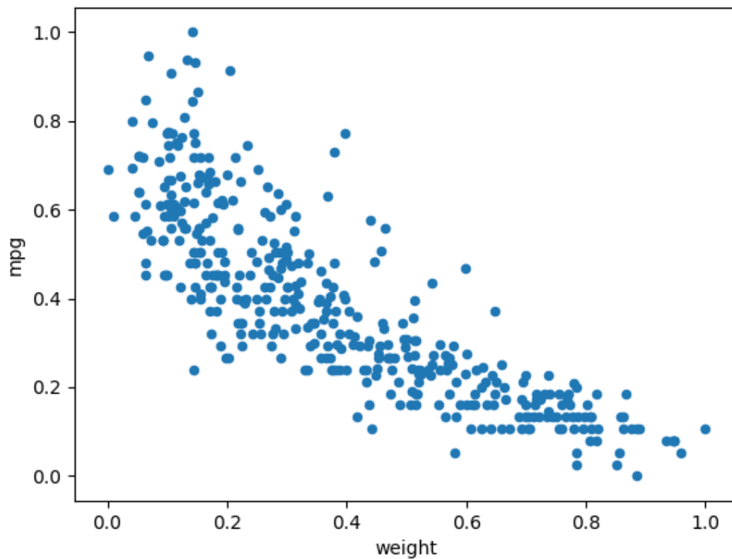
Figura 17: MPG Data
