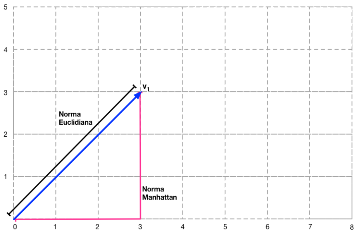
Figura 21: Norma L_1
