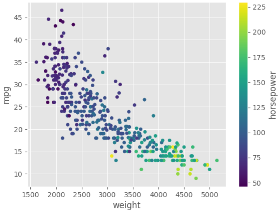
Figura 23: Plot con mapa de colores
