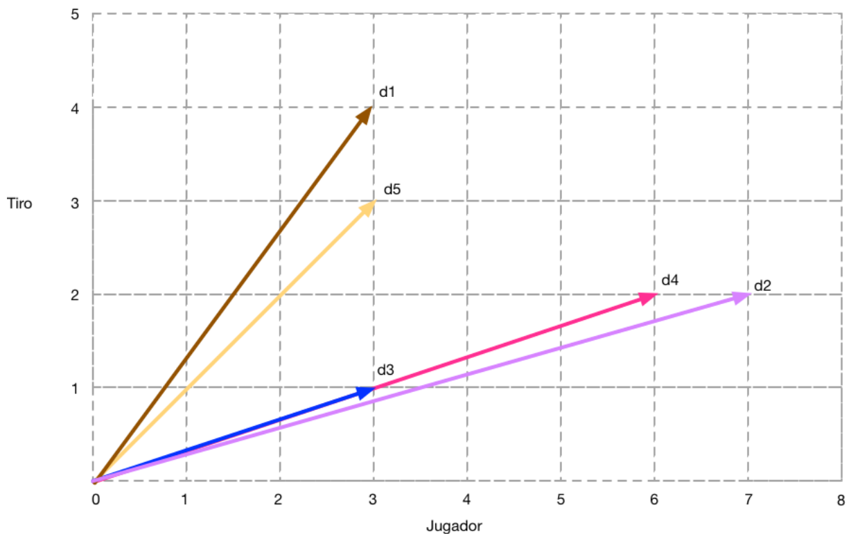
Figura 19: Vectores
