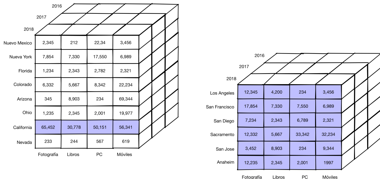
Figura 40: Operación Drill-Down
