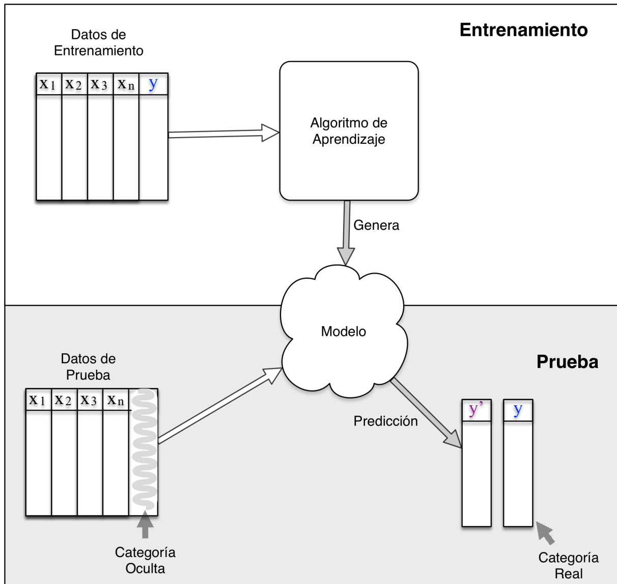
Figura 42: Aprendizaje supervisado
