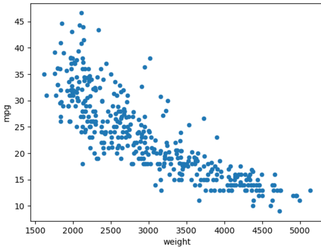
Figura 11: MPG Data
