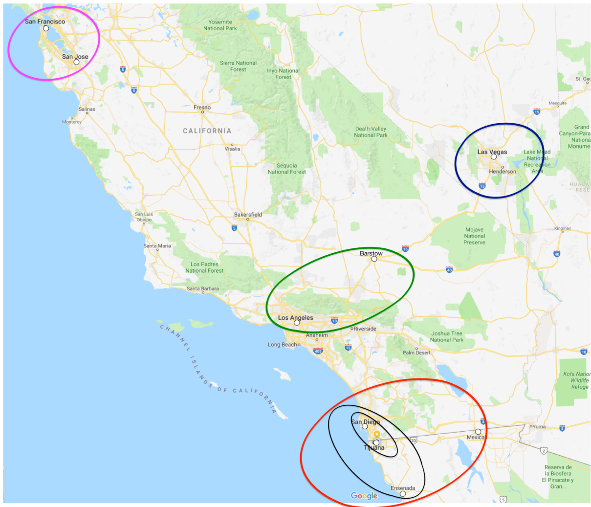
Figura 72: Agrupación jerárquica
