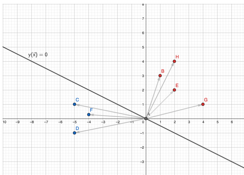
Figura 50: Objetos y función discriminante en 2D
