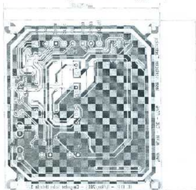
Fig 2.10 Circuito Cargador Solar
