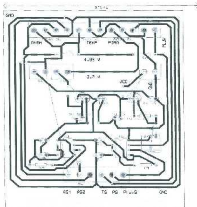
Fig 2.11 Circuito Fuente.
