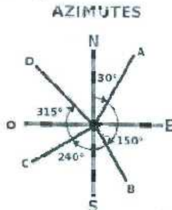
Fig 1.09 Representación Azimut.
