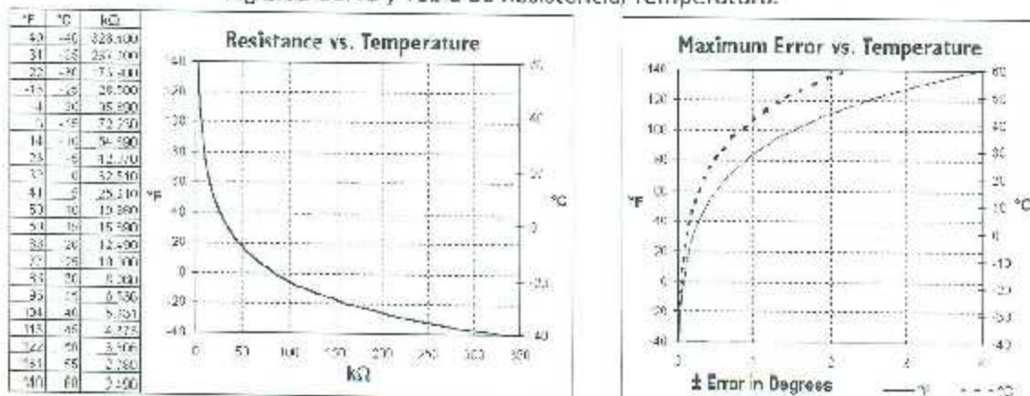
Fig 2.02 Curva y Tabla de Resistencia/Temperatura.
