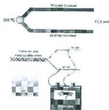
Fig 1.05 Termopar.
