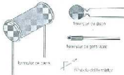
Fig 1.04 Termistores.
