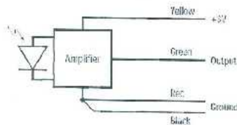
Fig 2.04 Diagrama Esquemático del Piranómetro.
