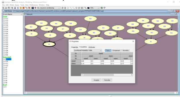
Figura 12. Probabilidades de un nodo interno (E1)
