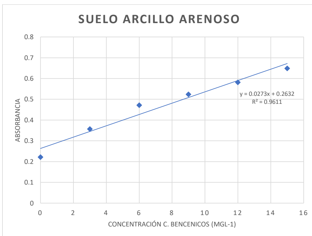
Figura 5.50. Curva de calibración para suelo Arcillo Arenoso.
