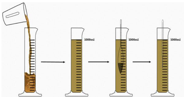
Figura 4.3. Diagrama del método del análisis textural de Bouyucos.
