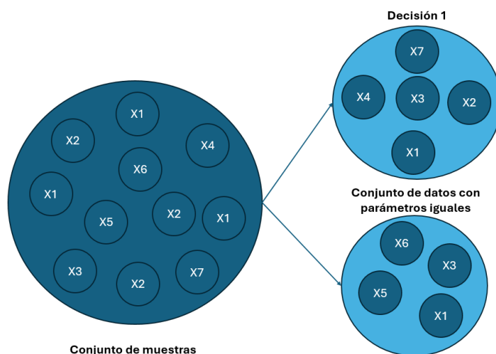
Figura 3.11. Principio del método Random Forest.
