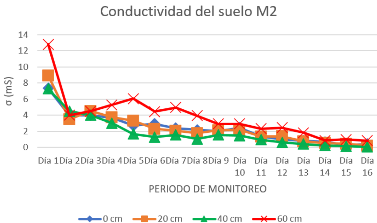
Figura 5.20. Tendencia de la conductividad en M2 contaminada.
