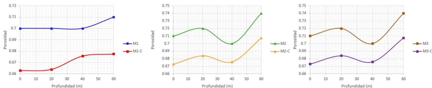
Figura 5.26. Comportamiento de la porosidad de suelo de las muestras M1, M2 y M3
