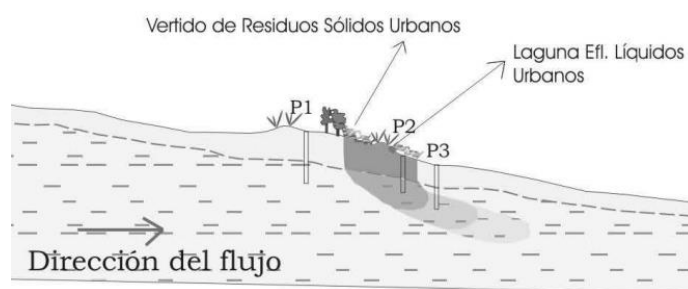
Figura 3.9. Diagrama del transporte por difusión (Gómez M, 2016).
