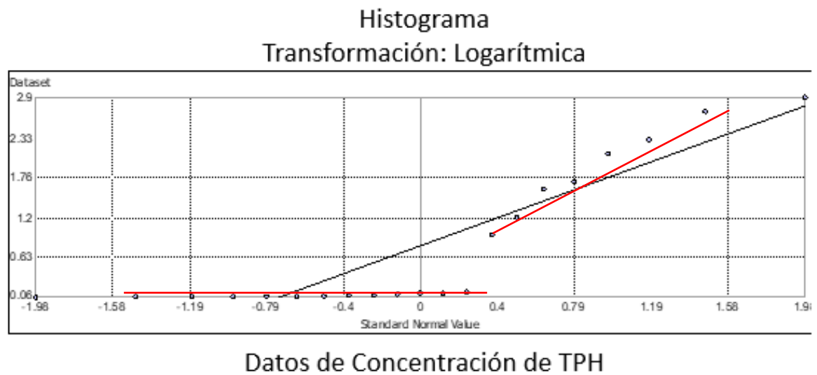
Figura 5.32. Gráfico de QQPLOT.
