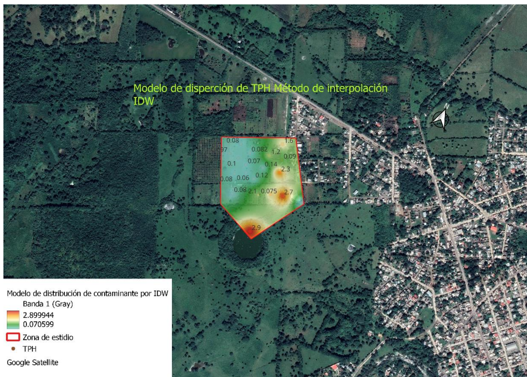
Figura 5.46. Distribución del contaminante método IDW.
