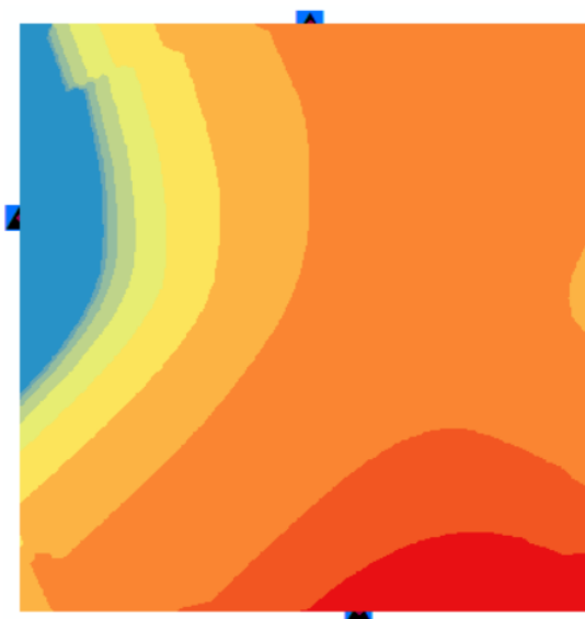
Figura 5.41. Modelo por método Interpolación Polinomial Local (IPL)
