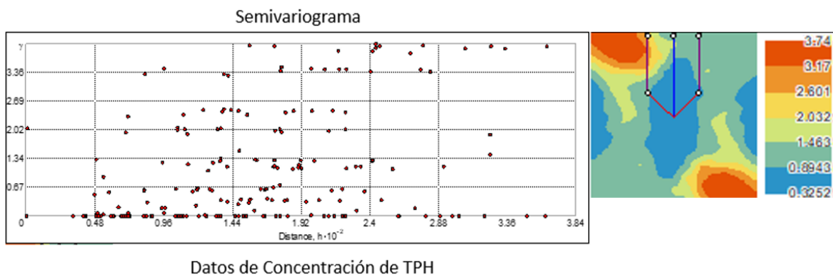
Figura 5.35. Varianza de la concentración de TPH
