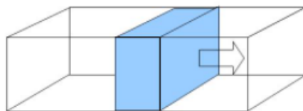
Figura 3.8. Diagrama del transporte por advección (flujo de soluto arrastrado por el fluido que pasa por una superficie).
