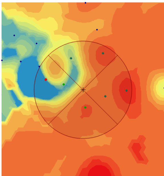
Figura 5.43. Modelo por el método de Kriging.
