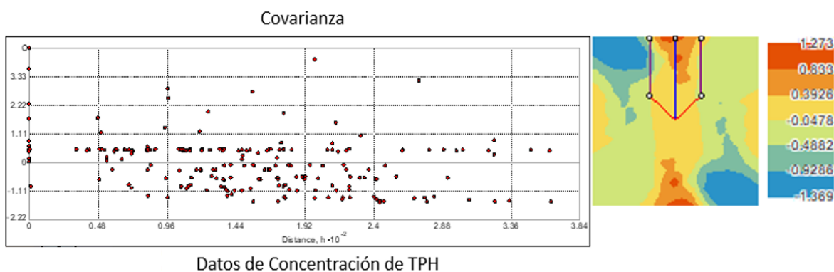
Figura 5.36. Covarianza de la concentración de TPH
