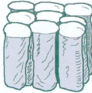
Figura 3.4. Estructura columnar.
