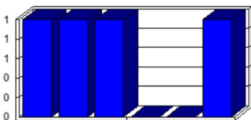
Figura 5.39. Distribución de la frecuencia IDW
