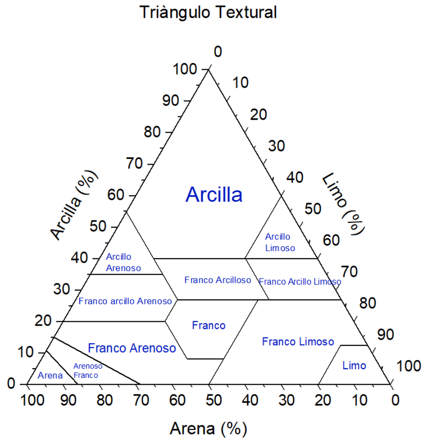
Figura 4.4. Triángulo textural de suelo (USDA).
