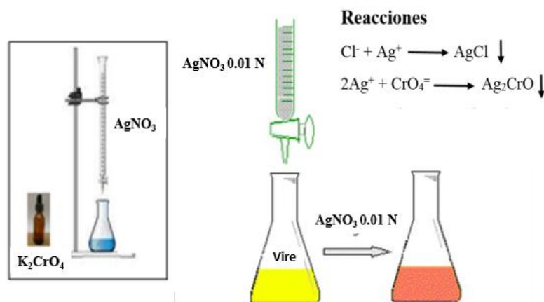
Figura 4.2. Diagrama del proceso de la técnica analítica de Mohr.
