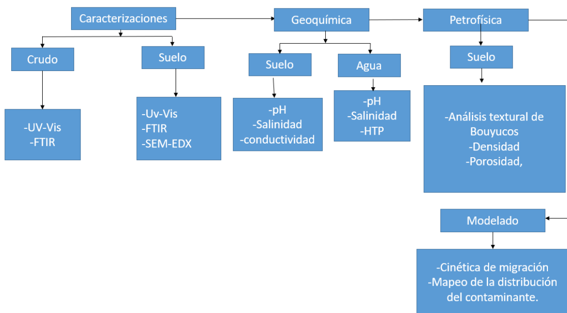
Figura 4.1. Diagrama de la metodología del proyecto.
