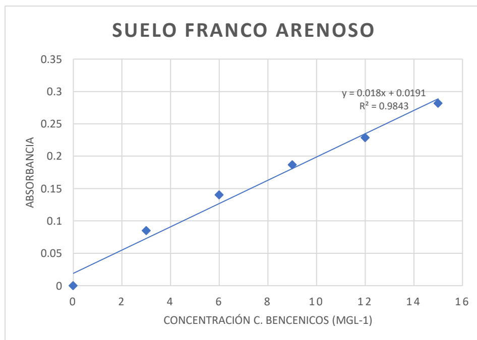
Figura 5.48. Curva de calibración para suelo Franco Arenoso.
