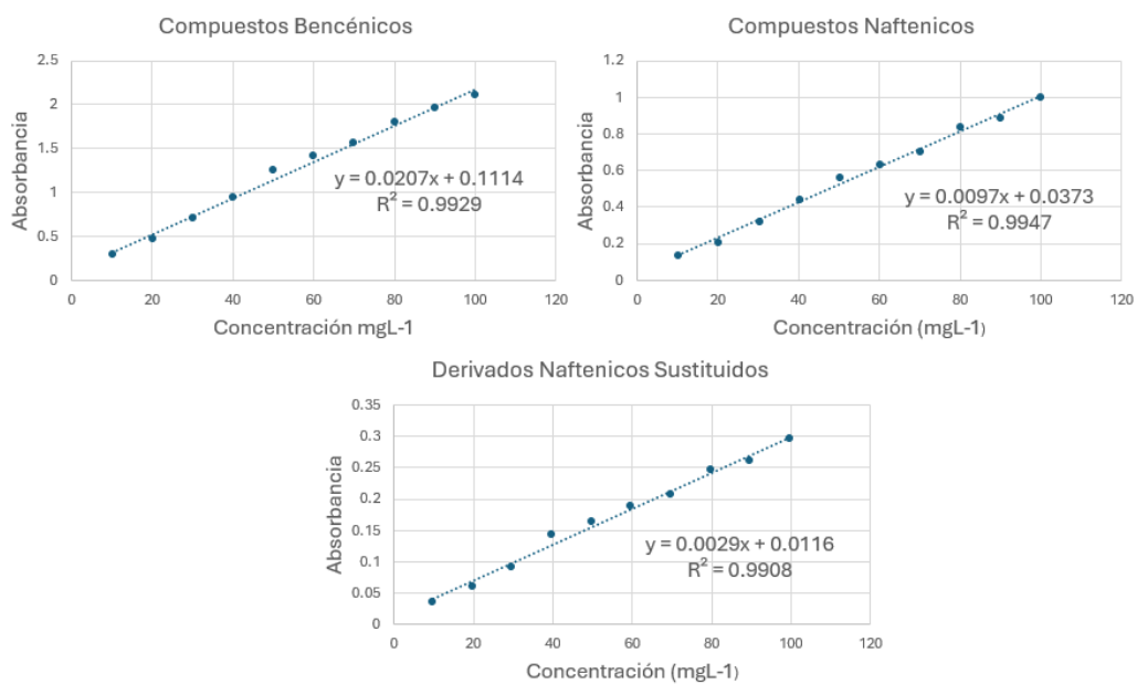
Figura 5.29. Curvas de calibración para cada compuesto contenido en el crudo Aragón.
