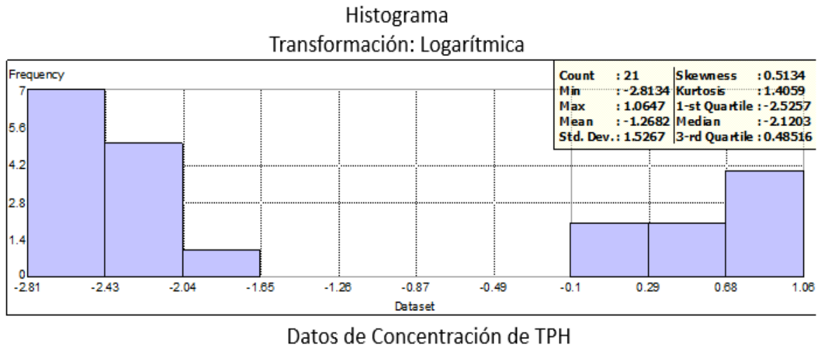
Figura 5.31. Histograma (campana Gaussiana).
