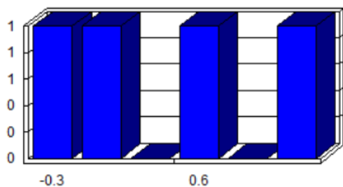
Figura 5.38. Distribución de frecuencia IPL
