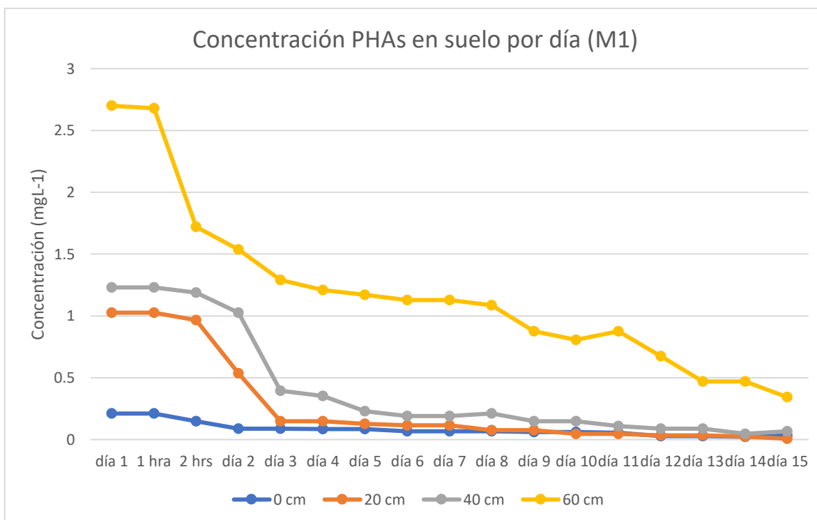
Figura 5.51. Concentración de contaminación de la muestra M1.
