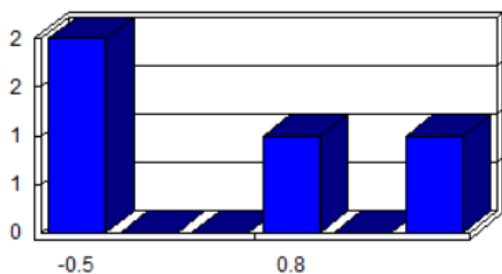
Figura 5.40. Distribución de la frecuencia
