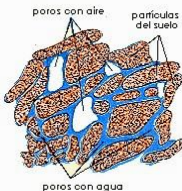
Figura 3.1. Diagrama de la fase líquida y gaseosa del suelo.
