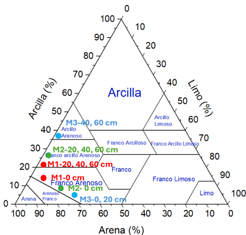
Figura 5.8. Clasificación el suelo en el triángulo textural (USDA).
