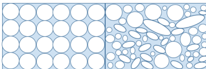
Figura 3.6. Representación de la porosidad de un material.
