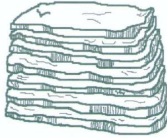
Figura 3.3. Estructura laminar.
