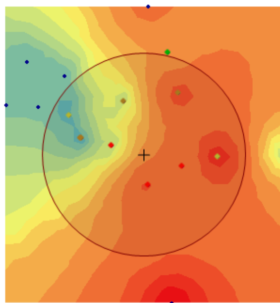
Figura 5.42. Modelo por el método de Distancia Inversa Ponderada (IDW)
