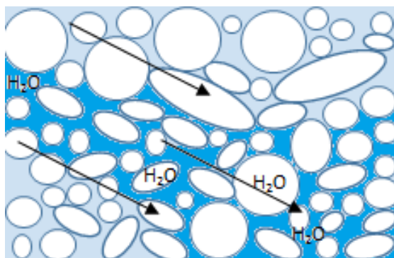
Figura 3.7. Representación de la permeabilidad.
