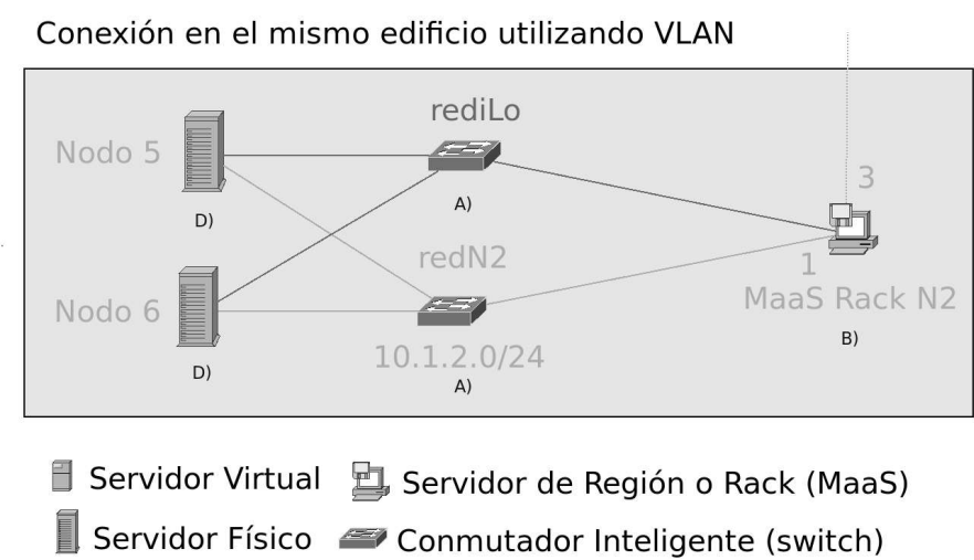
Figura 4.4: Diagrama de conexión en el mismo edificio utilizando VLAN.
