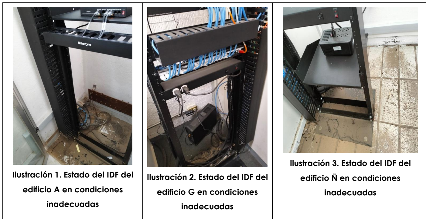
Figura 5.1 – Evidencia del estado físico deteriorado de los racks de comunicaciones.
