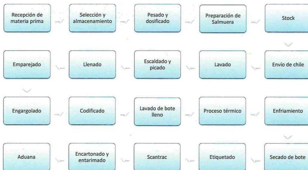
Ilustración 15. Diagrama general de proceso.
