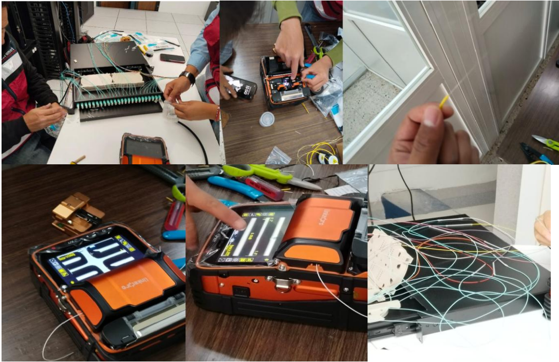
Figura 11 Proceso de fusión de fibra óptica.
