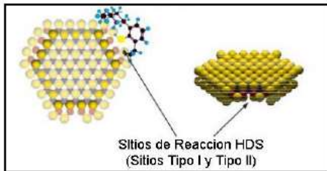
Figura 2.6. Sitios de Reacción HDS de Co (Ni)-Mo-S Tipo I y Tipo II.
